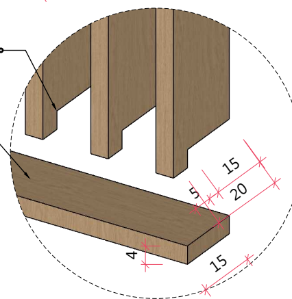
• Detalhe Ripado Esc.: 1/10
