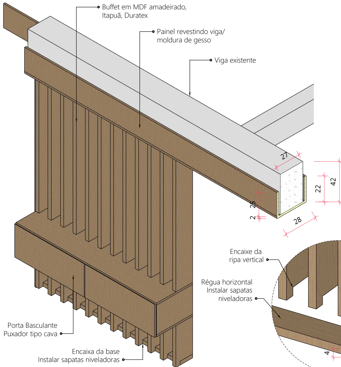
• Perspectiva Buffet Esc.: 1/20
