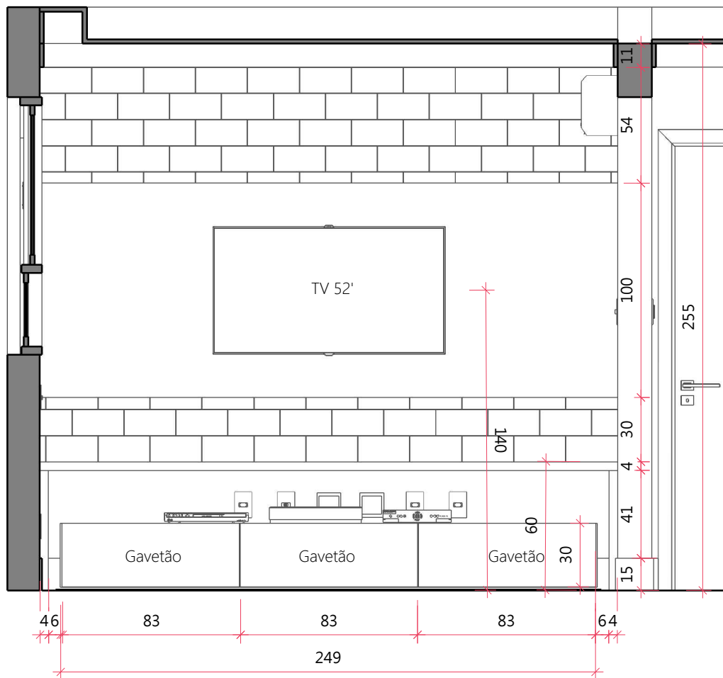
Vista A- Técnico Esc.: 1/25
