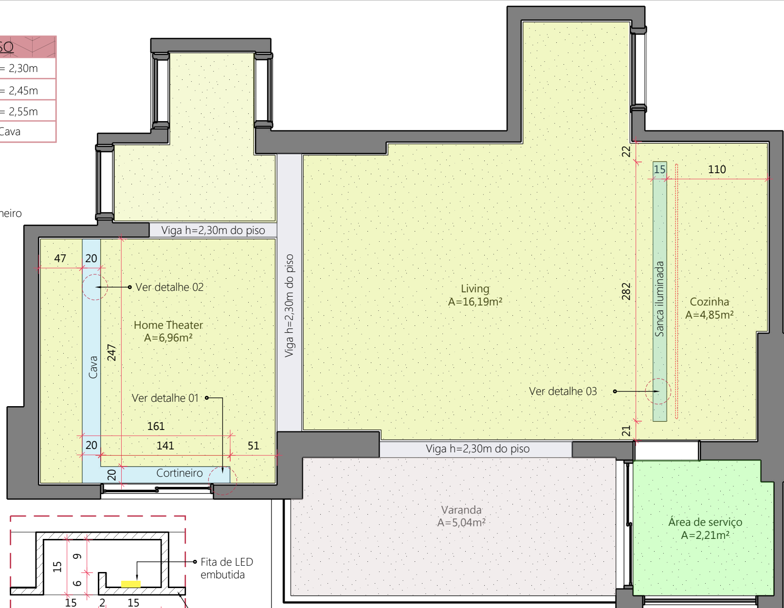
● Planta de Forro- Sala ampliada Esc.: 1/40
