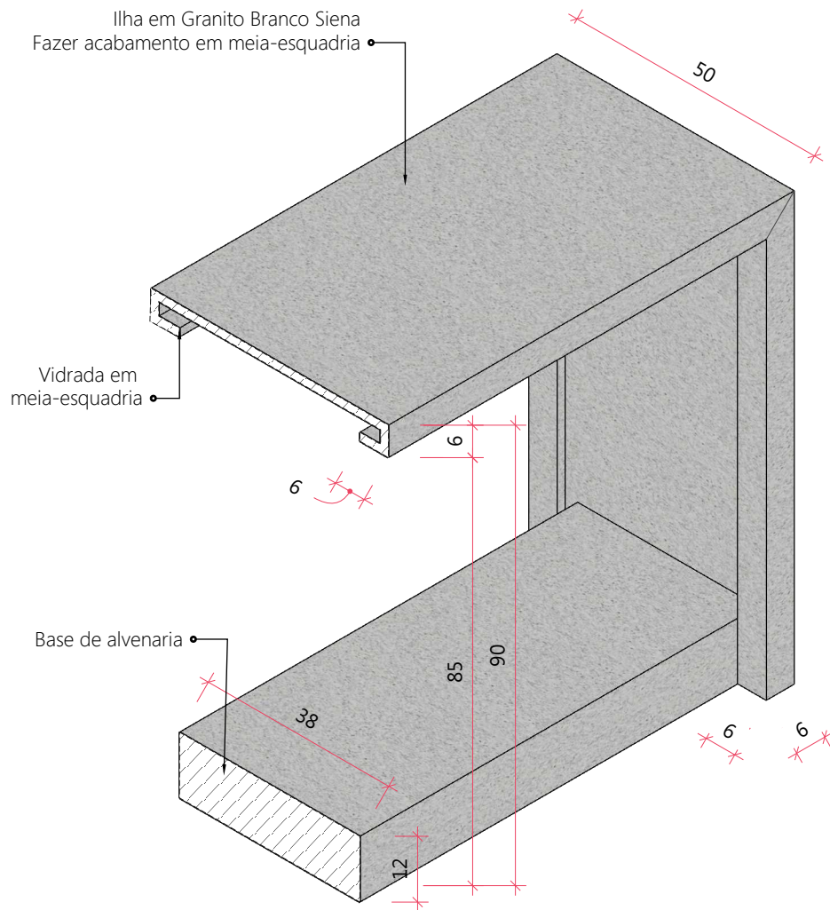
● Detalhe Marmoraria Esc.: 1/10
