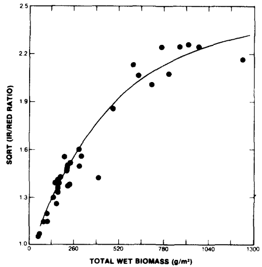
(d) r^2 = 0.89 Y = 2.4 - \exp(0.3926 - 0.00022 \cdot X)
