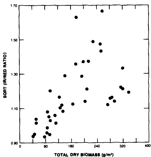
(d) r^2 = 0.36
