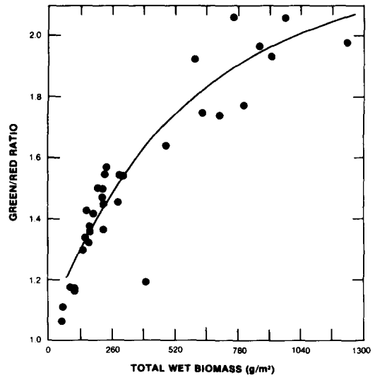
(d) r^2=0.82 Y=2.2-\exp(0.1081-0.0012 \cdot X) June data
