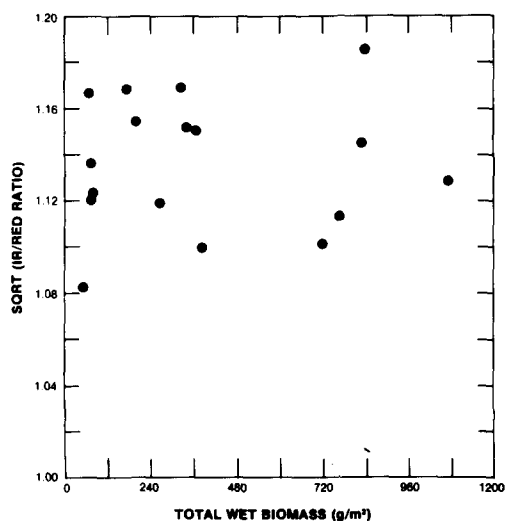
(d) r^2=0.00
