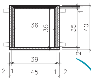
CORTE
