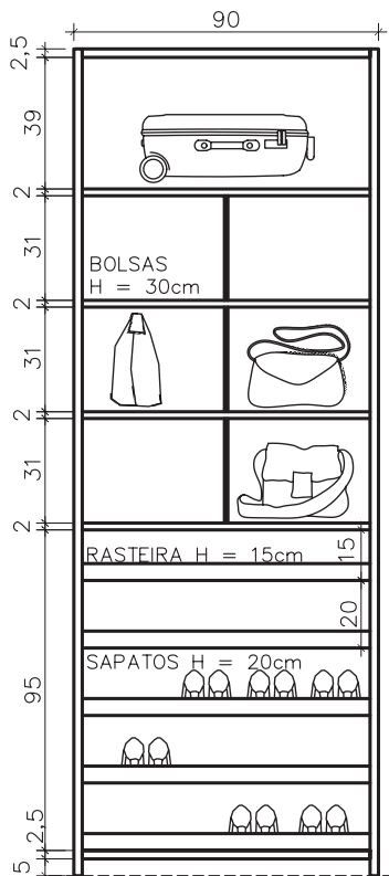
VISTA ARMÁRIO ACESSÓRIOS
