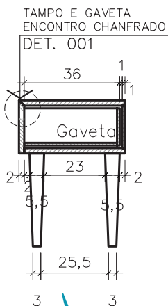
CORTE
