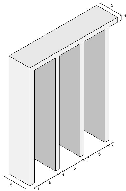
DETALHE GRADIL METÁLICO SEM ESCALA
