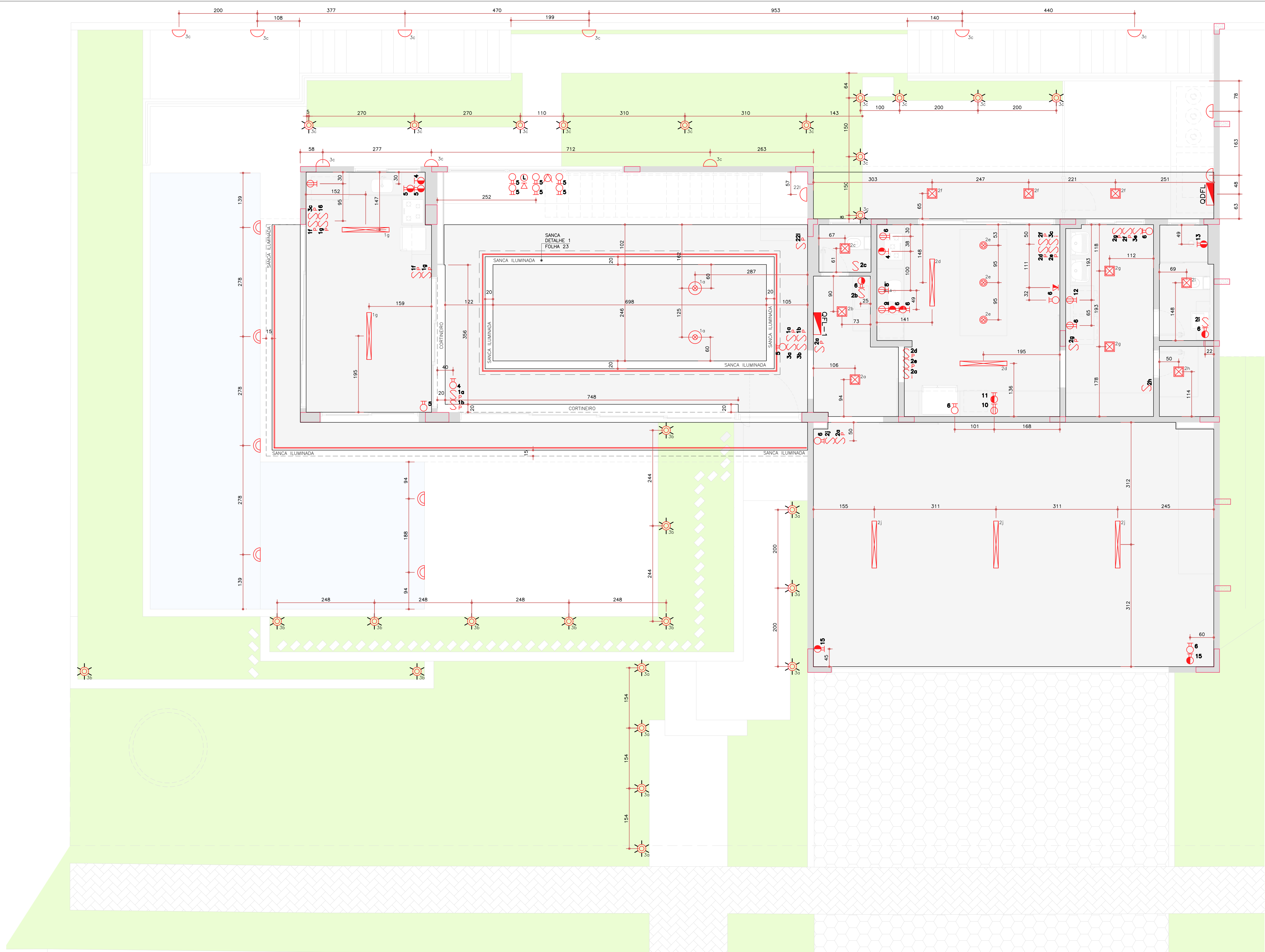
PLANTA PONTOS DE ILUMINAÇÃO – PAV. TÉRREO
