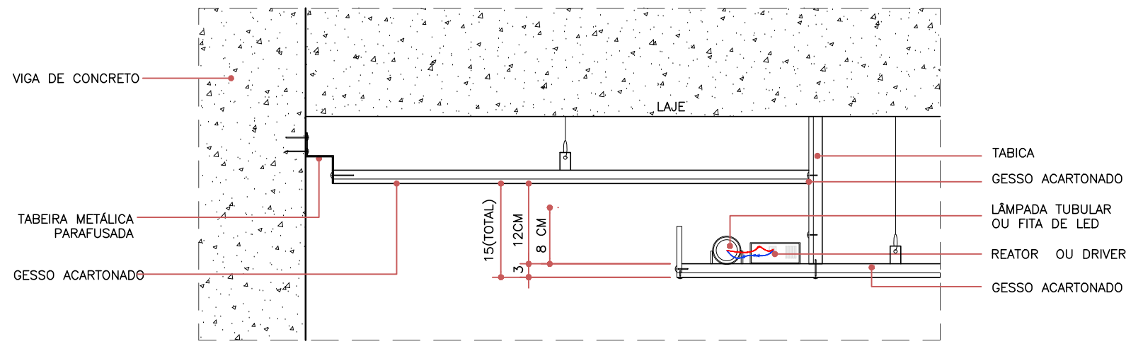
DET-02 SANCA DE GESSO COM ILUMINAÇÃO – SUITE MASTER
