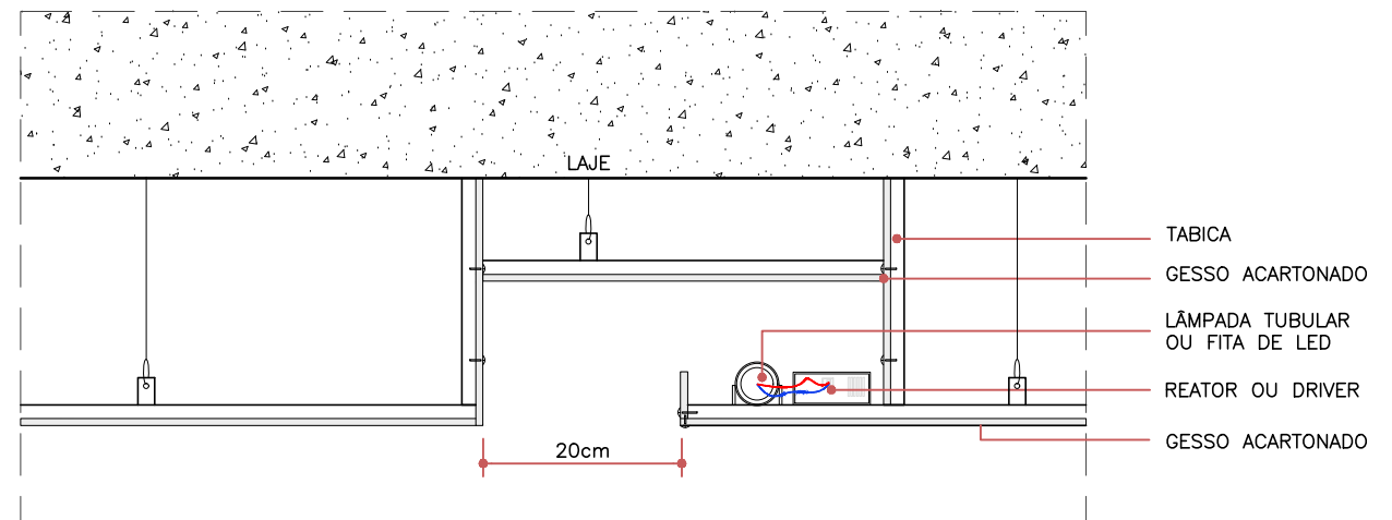
DET-01 SANCA DE GESSO COM ILUMINAÇÃO – SALA DE ESTAR
