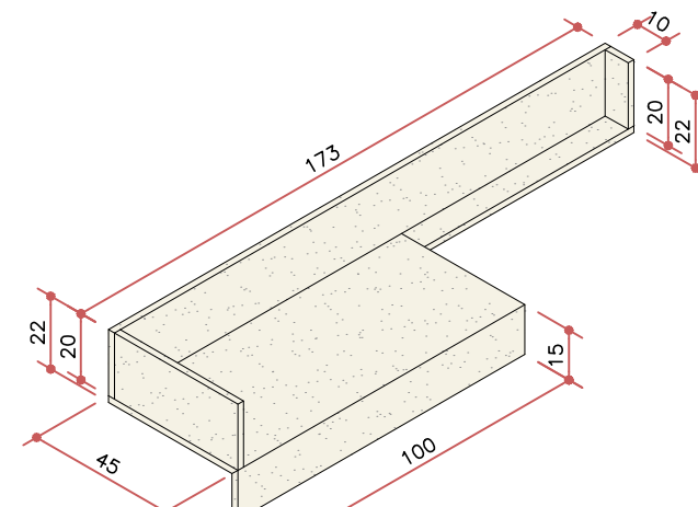
BANHO 3 - MARMORARIA ESC. 1:25 obs: conferir medidas na obra.
