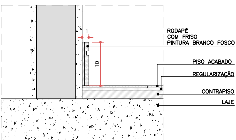
DET. RODAPÉ 2 DE MDF
