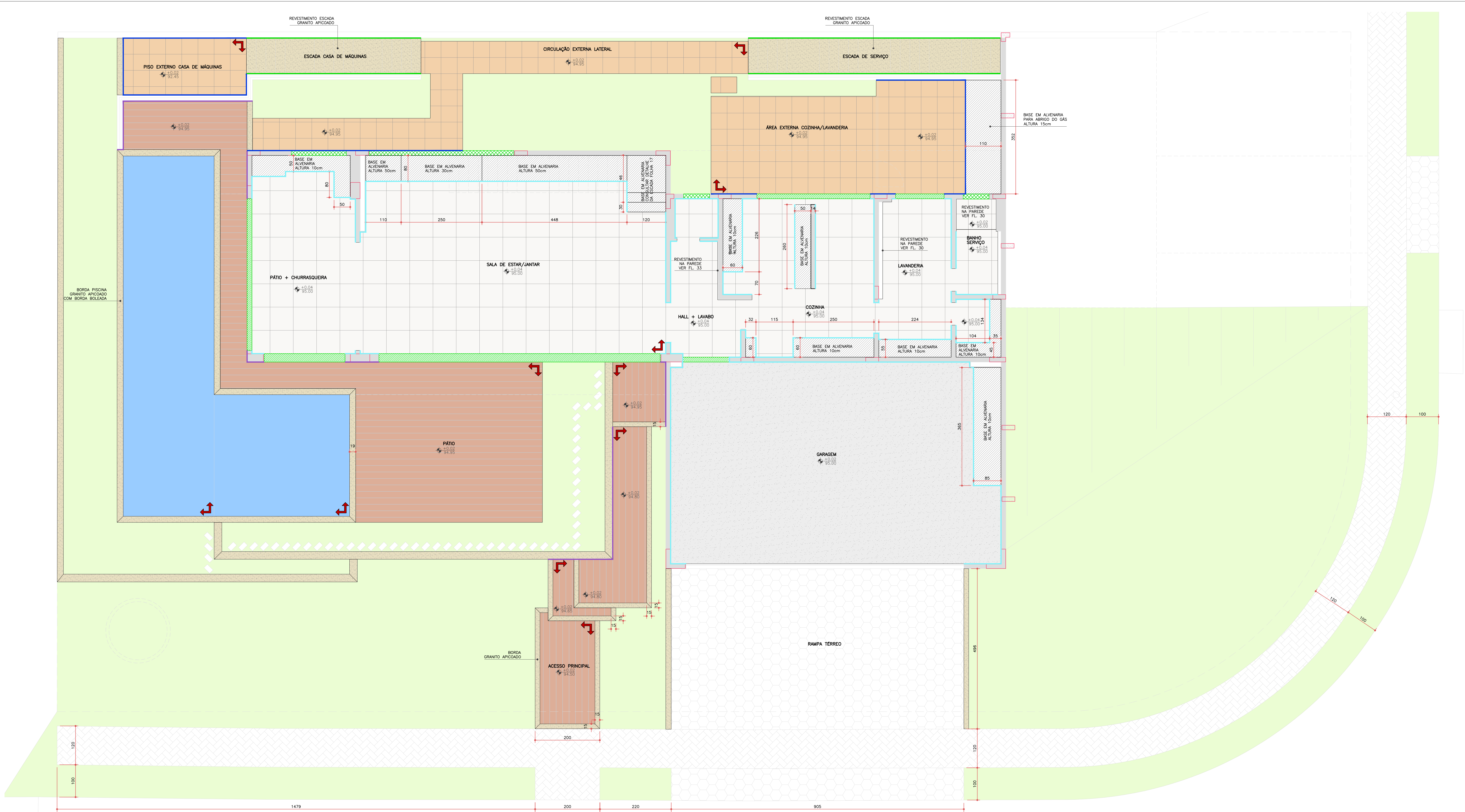
PLANTA DE PISO – PAV. TERREO ESC. 1:50
