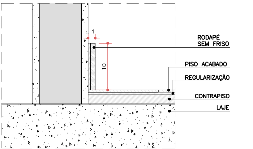
DET. RODAPÉ 1 DE PORCELANATO
