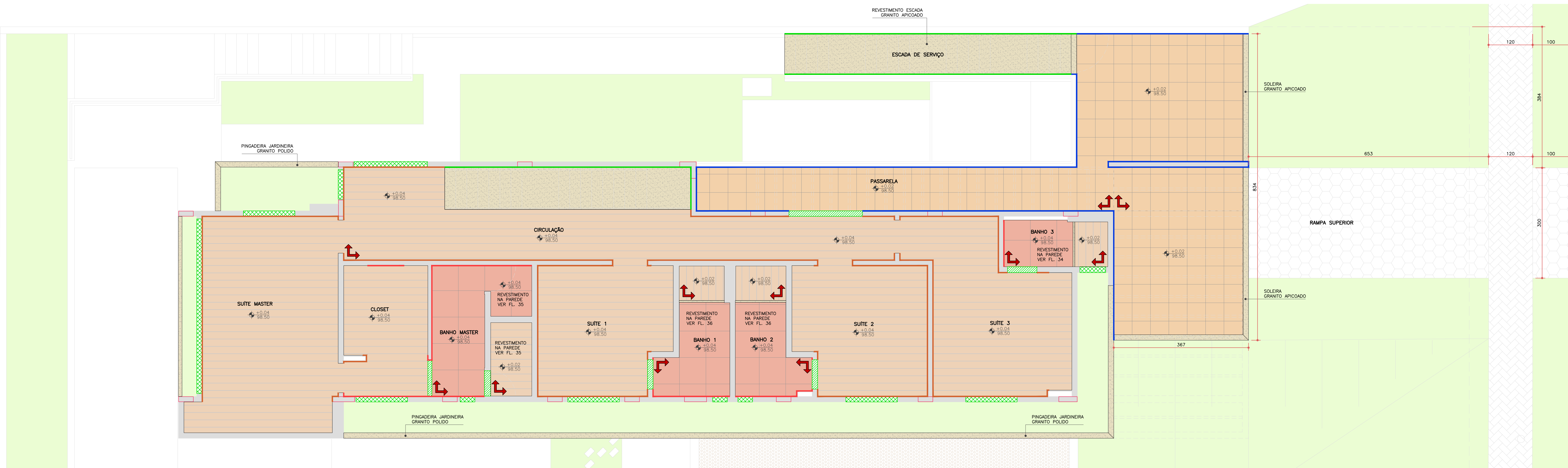
PLANTA DE PISO – PAV. SUPERIOR ESC. 1:50
