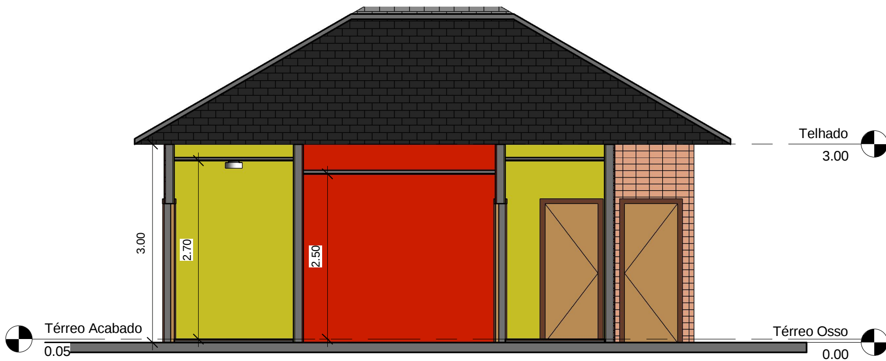
1 Corte 1 : 50
