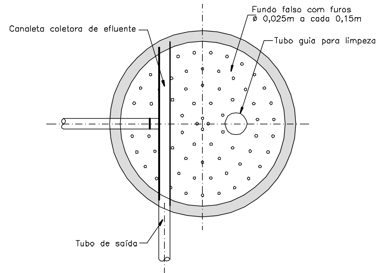
PLANTA BAIXA C-C FILTRO ANAERÓBICO
