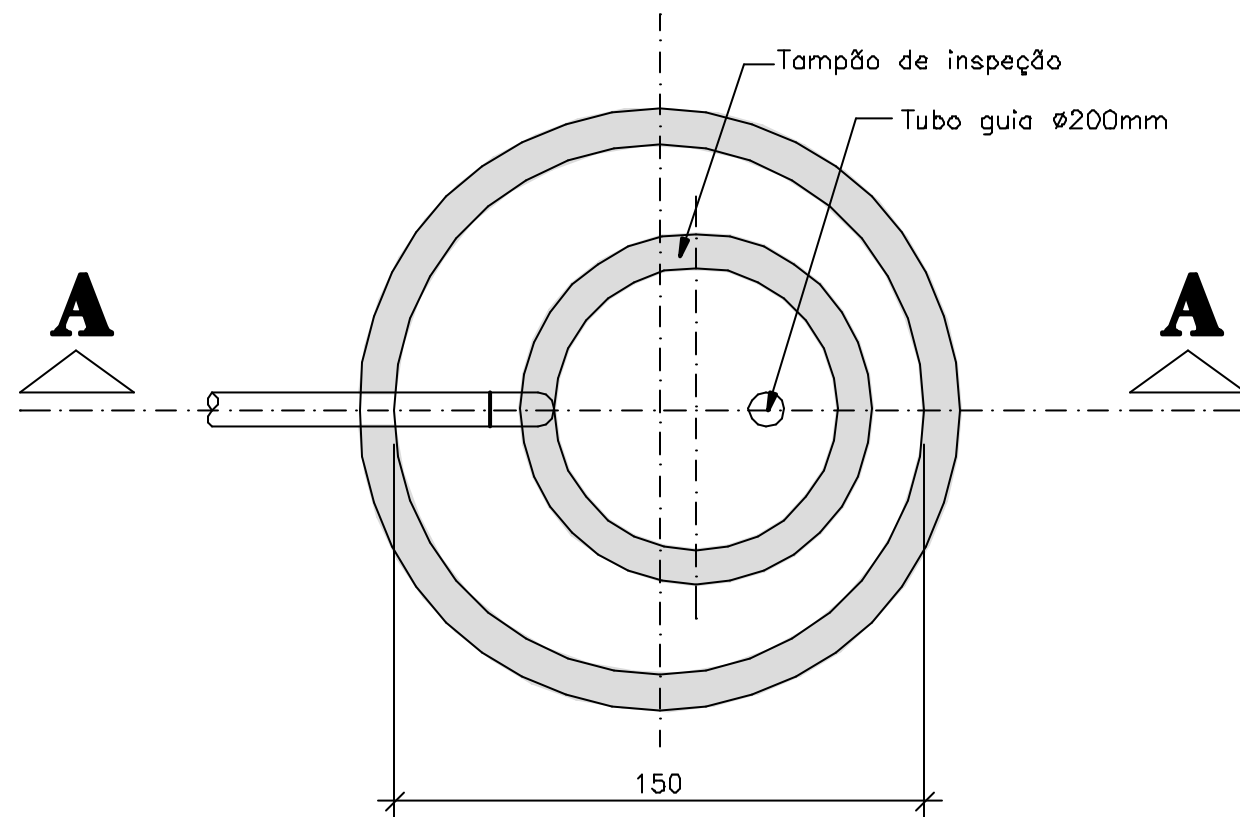
PLANTA BAIXA B-B FILTRO ANAERÓBICO
