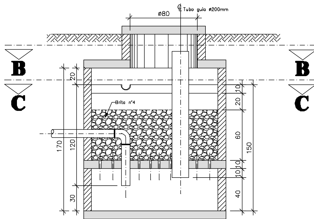
CORTE AA-FILTRO ANAERÓBIO
