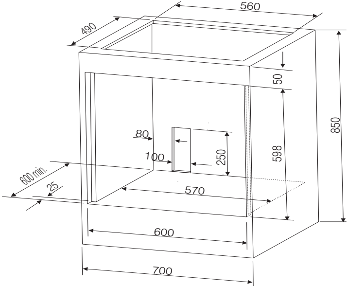
Figura 2.0 - dimensões em mm
