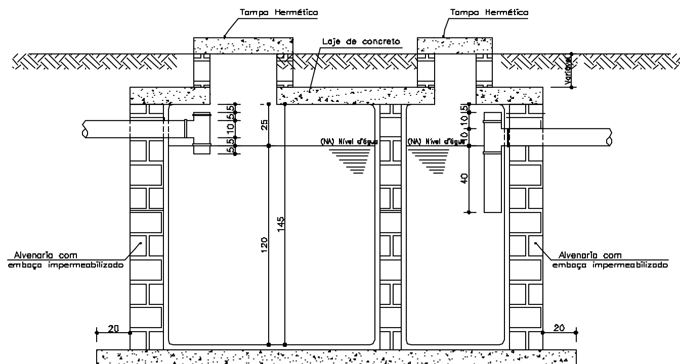
CORTE AA—TANQUE SÉPTICO
