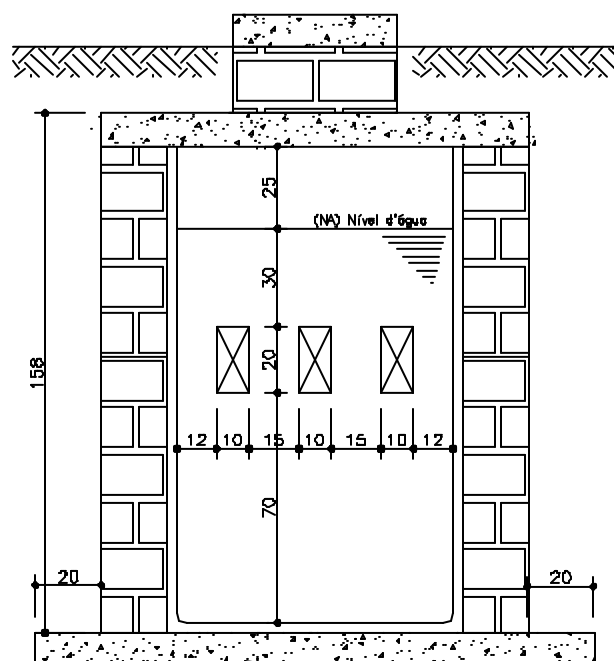
CORTE BB—TANQUE SÉPTICO
