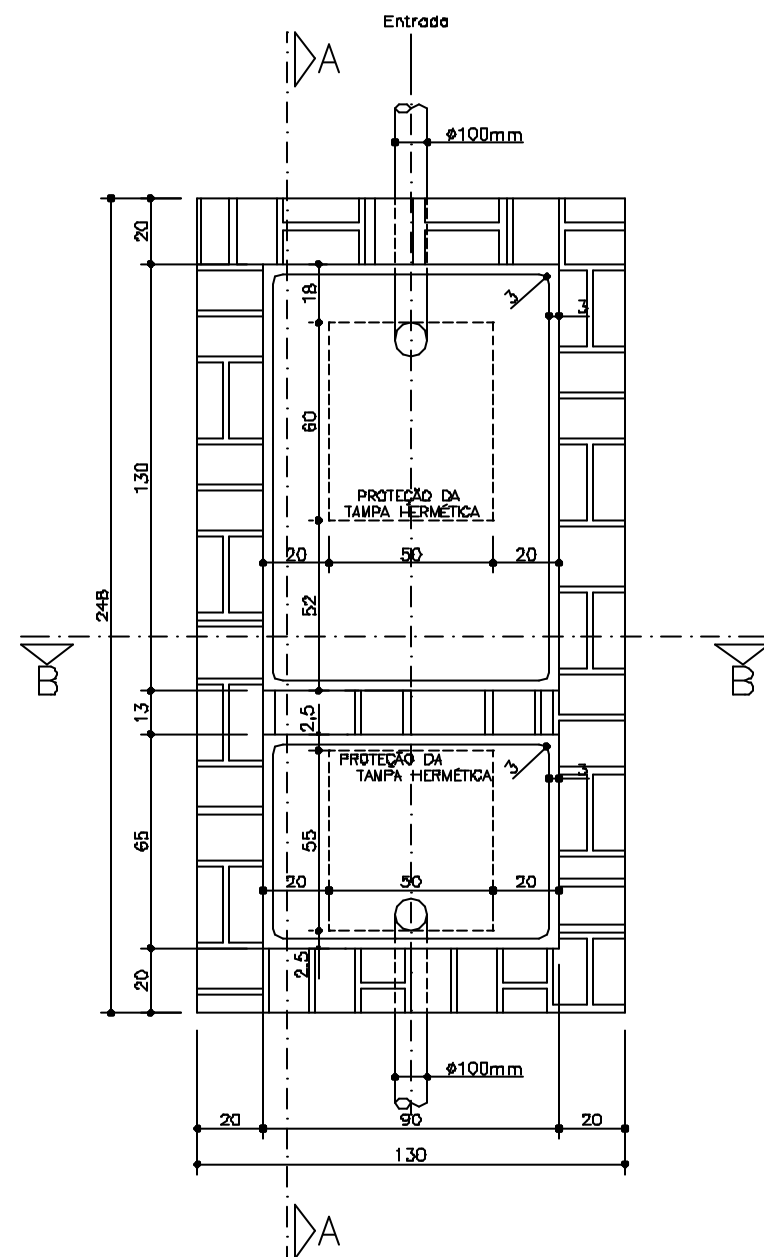
PLANTA BAIXA—TANQUE SÉPTICO
