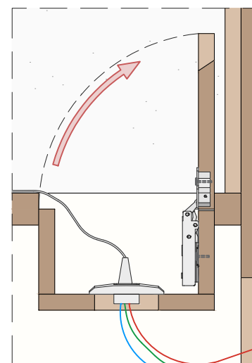
DET. CORTE - ABERTURA ESC. 1:5
