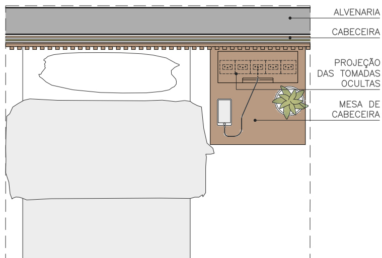
PLANTA ESC. 1:20
