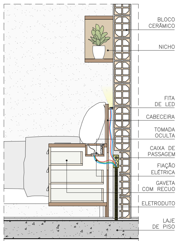
CORTE ESC. 1:20
