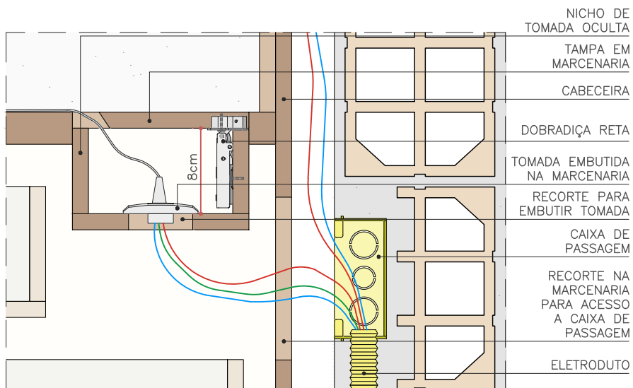
DET. CORTE ESC. 1:5
