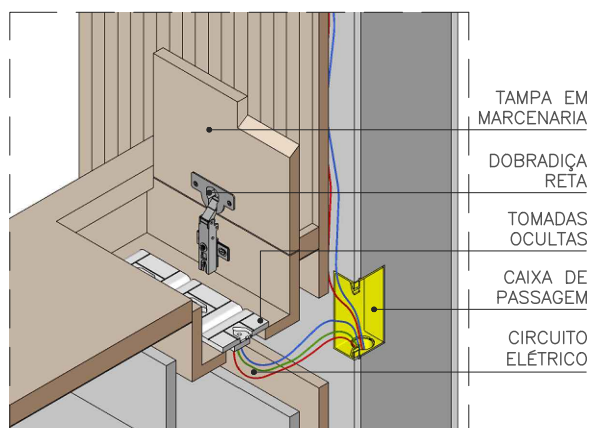
ISOMÉTRICA - ABERTO SEM ESCALA
