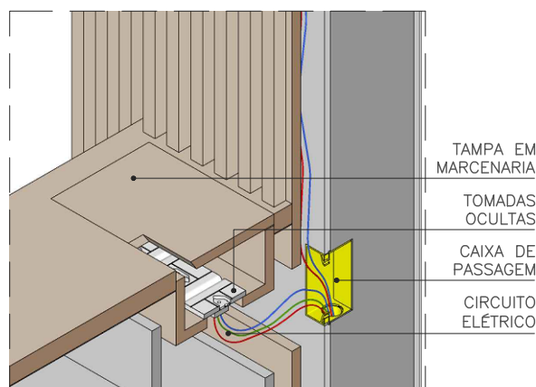
ISOMÉTRICA - FECHADO SEM ESCALA
