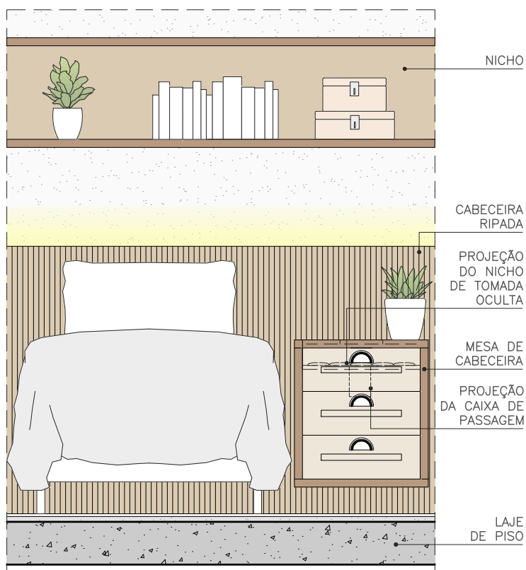
VISTA FRONTAL ESC. 1:20
