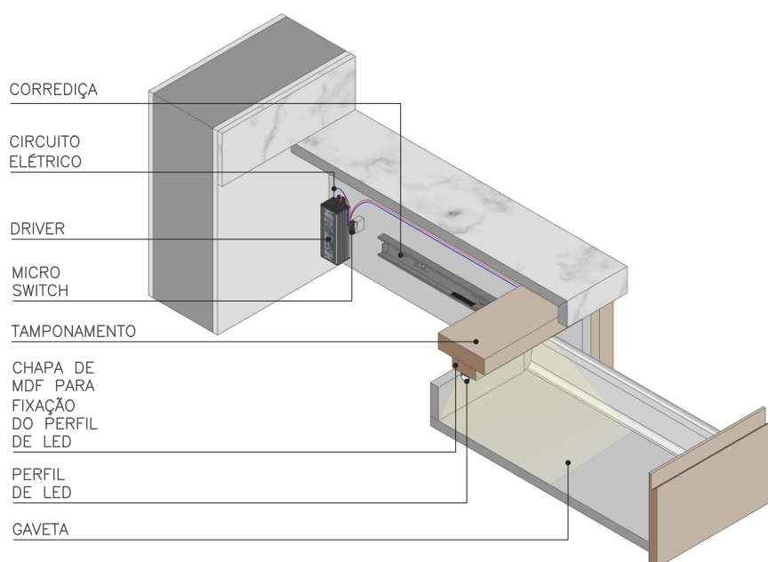
ISOMÉTRICA - GAVETA ABERTA SEM ESCALA
