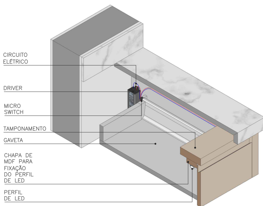
ISOMÉTRICA - GAVETA FECHADA SEM ESCALA
