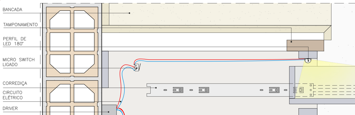
DET. LED LIGADO ESC. 1:5
