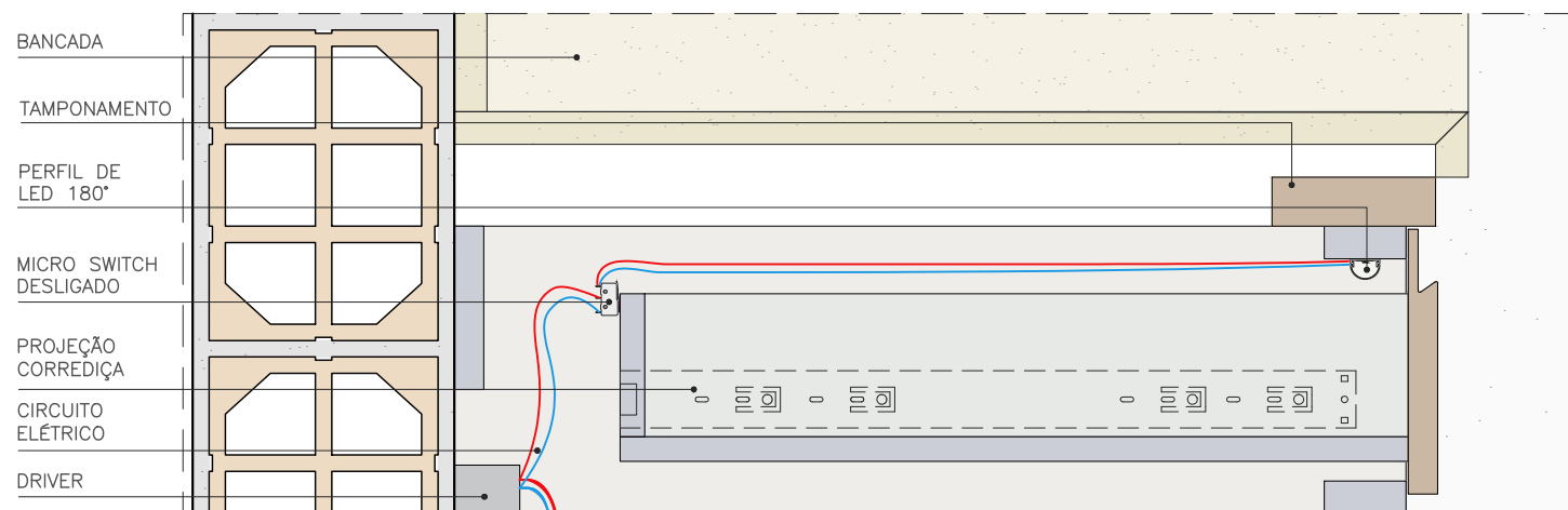
DET. LED DESLIGADO ESC. 1:5
