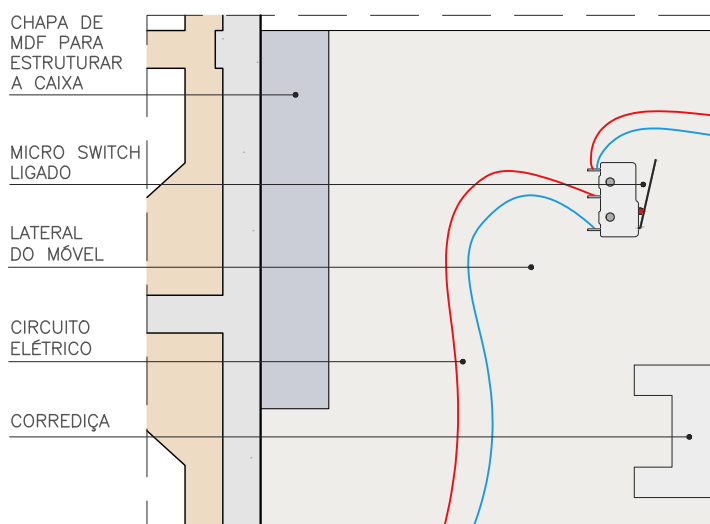
DET. SWITCH LIGADO ESC. 1:2
