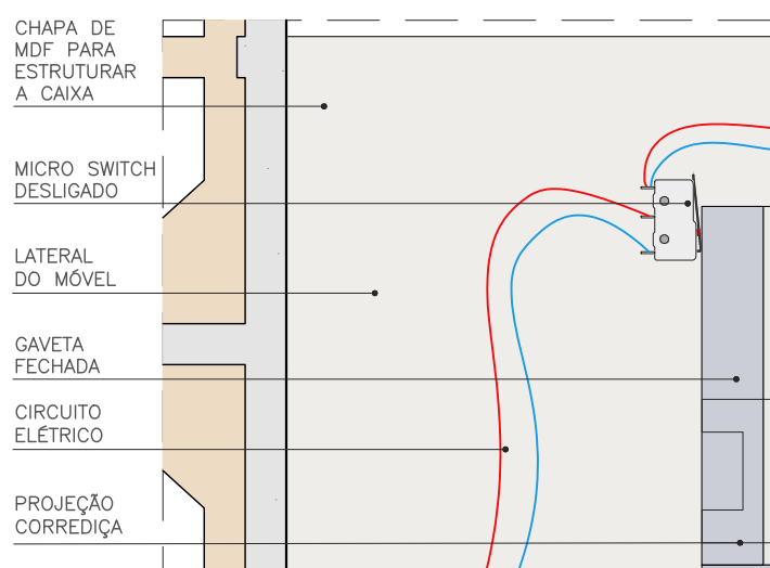
DET. SWITCH DESLIGADO ESC. 1:2
