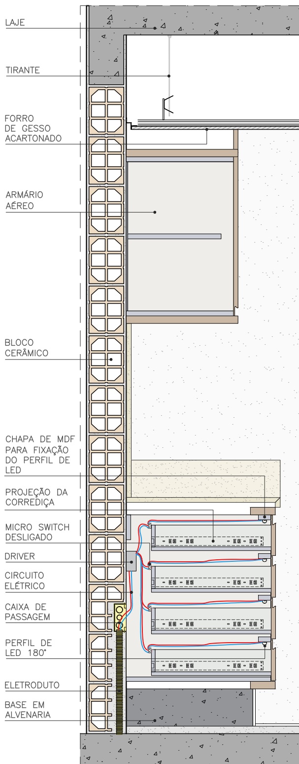
CORTE GERAL ESC. 1:20
