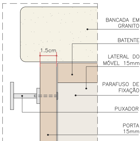
INFERIORES ESC. 1:2
