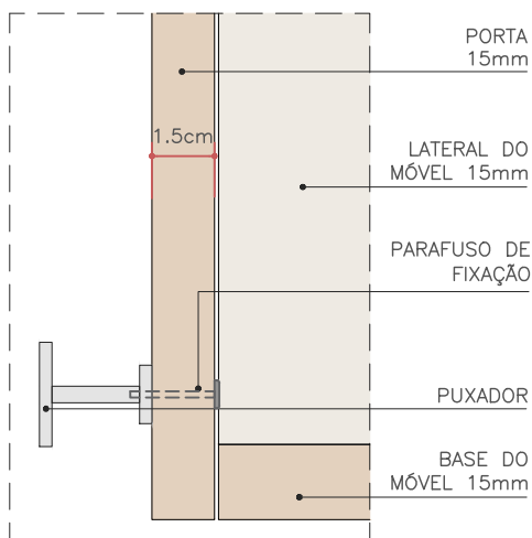
SUPERIORES ESC. 1:2
