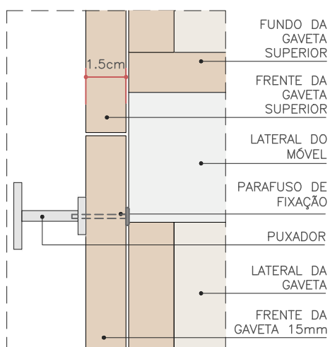
GAVETEIRO ESC. 1:2
