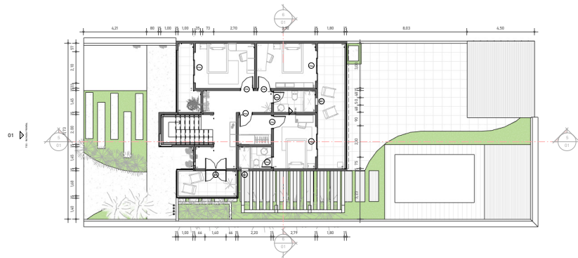
002 TEC - SUPERIOR 1:100
