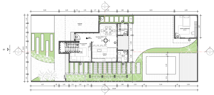
001 TEC - TÉRREO 1:100
