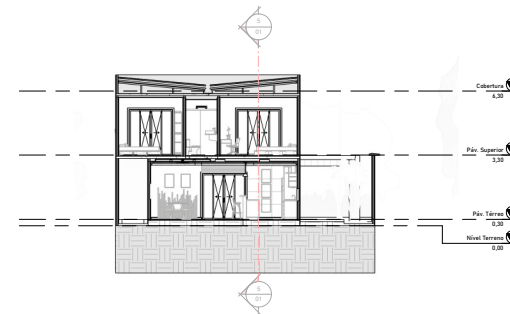
006 TEC - CORTE BB 1:100
