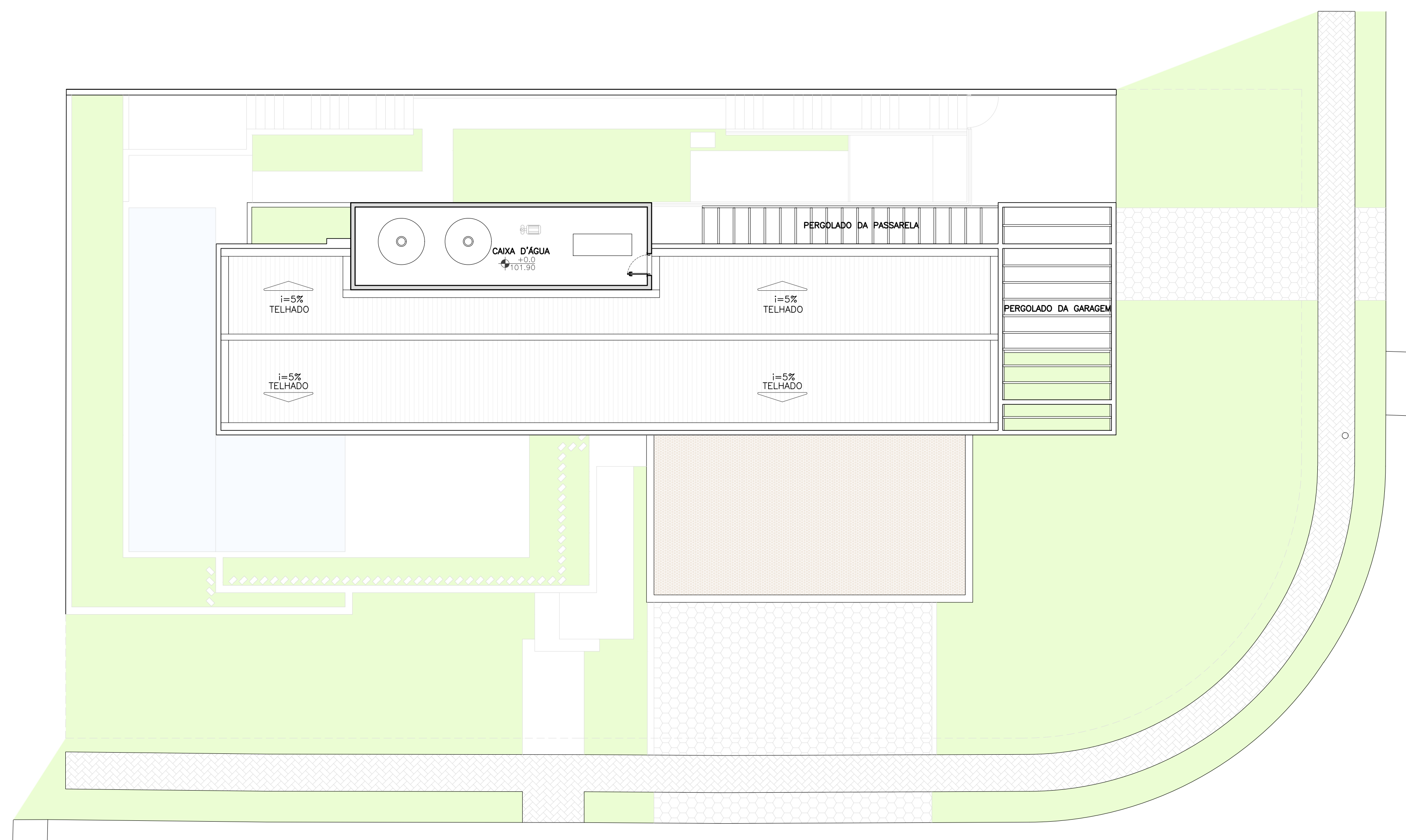
LAYOUT - CAIXA D'ÁGUA 1:100
