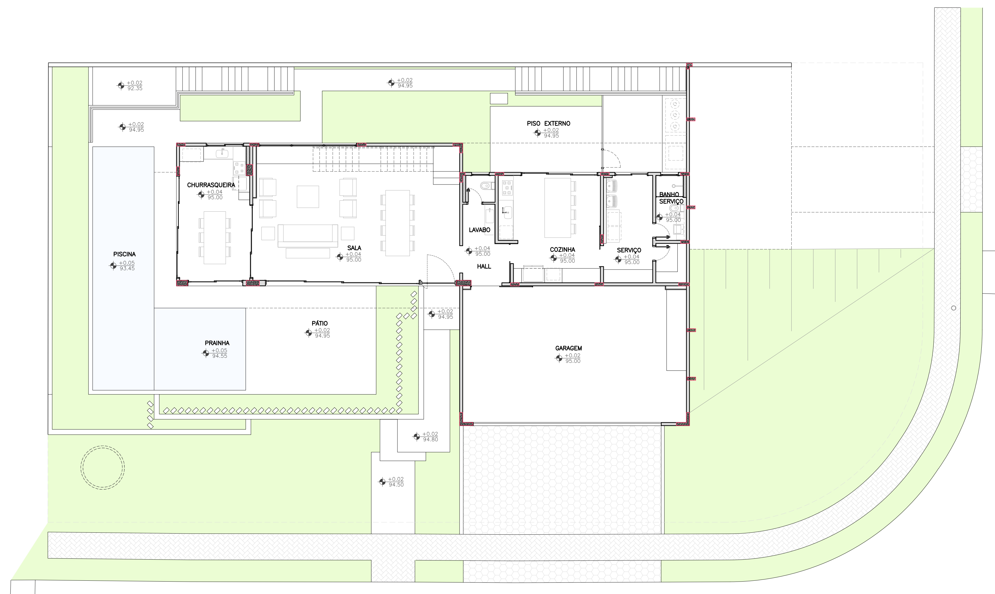
LAYOUT - PAV. TÉRREO 1:100
