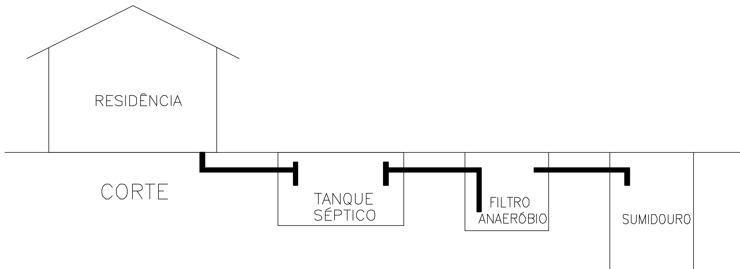
SISTEMA LOCAL DE TRATAMENTO DE ESGOTO – IMPLANTAÇÃO
