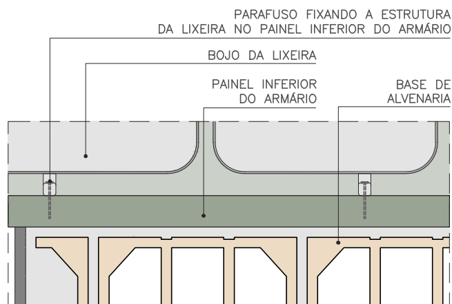
DETALHE - FIXAÇÃO - CORTE ESC. 1:5
