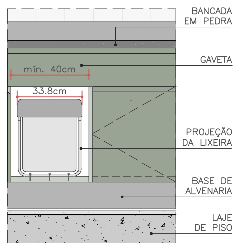
VISTA FRONTAL ESC. 1:20
