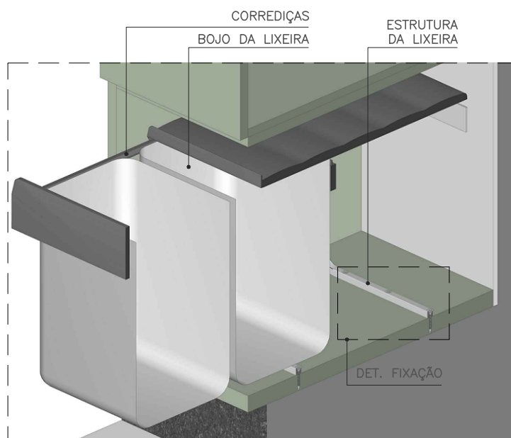
ISOMÉTRICA - DET LIXEIRA SEM ESCALA
