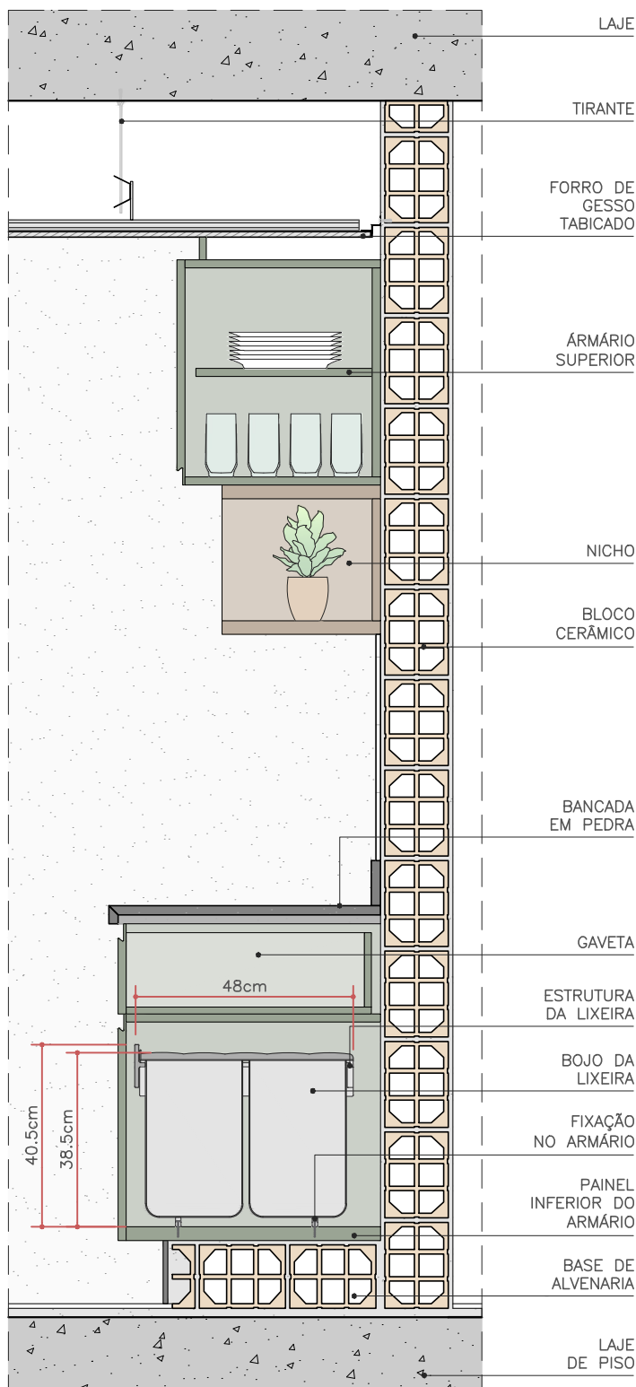
CORTE - LIXEIRA FECHADA ESC. 1:15
