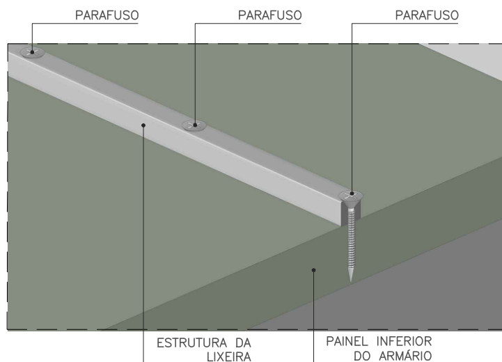
ISOMÉTRICA - DET. FIXAÇÃO SEM ESCALA
