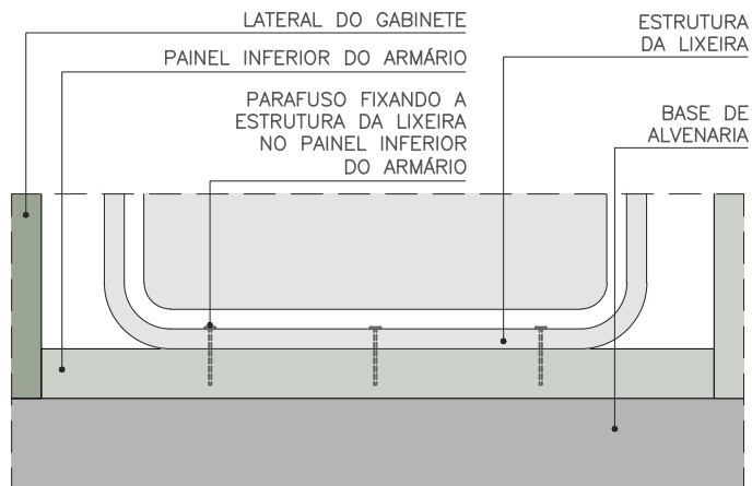
DETALHE - FIXAÇÃO - VISTA FRONTAL ESC. 1:5
