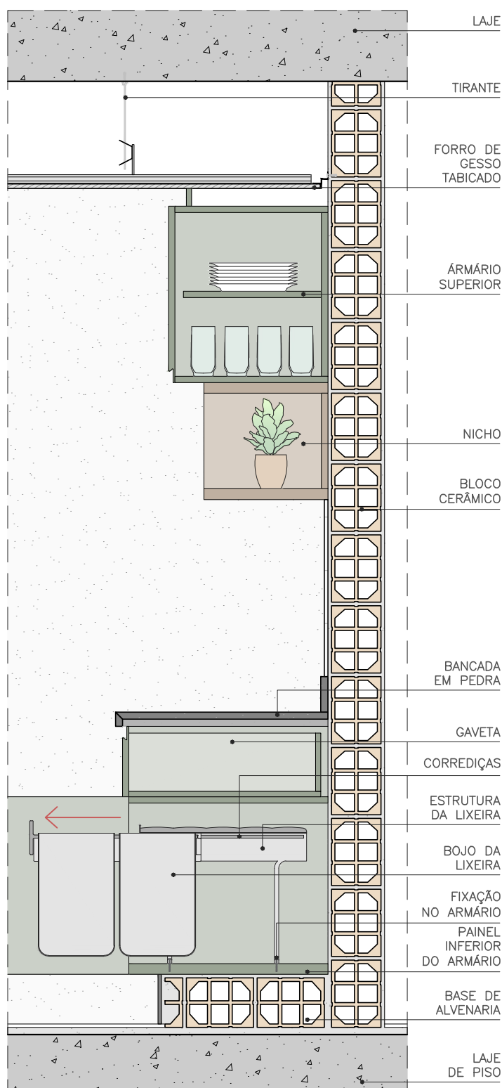
CORTE - LIXEIRA ABERTA ESC. 1:15
