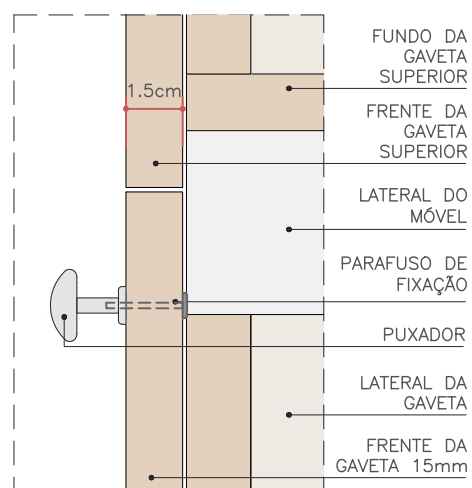
GAVETEIRO ESC. 1:2
