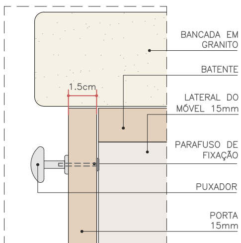
INFERIORES ESC. 1:2
