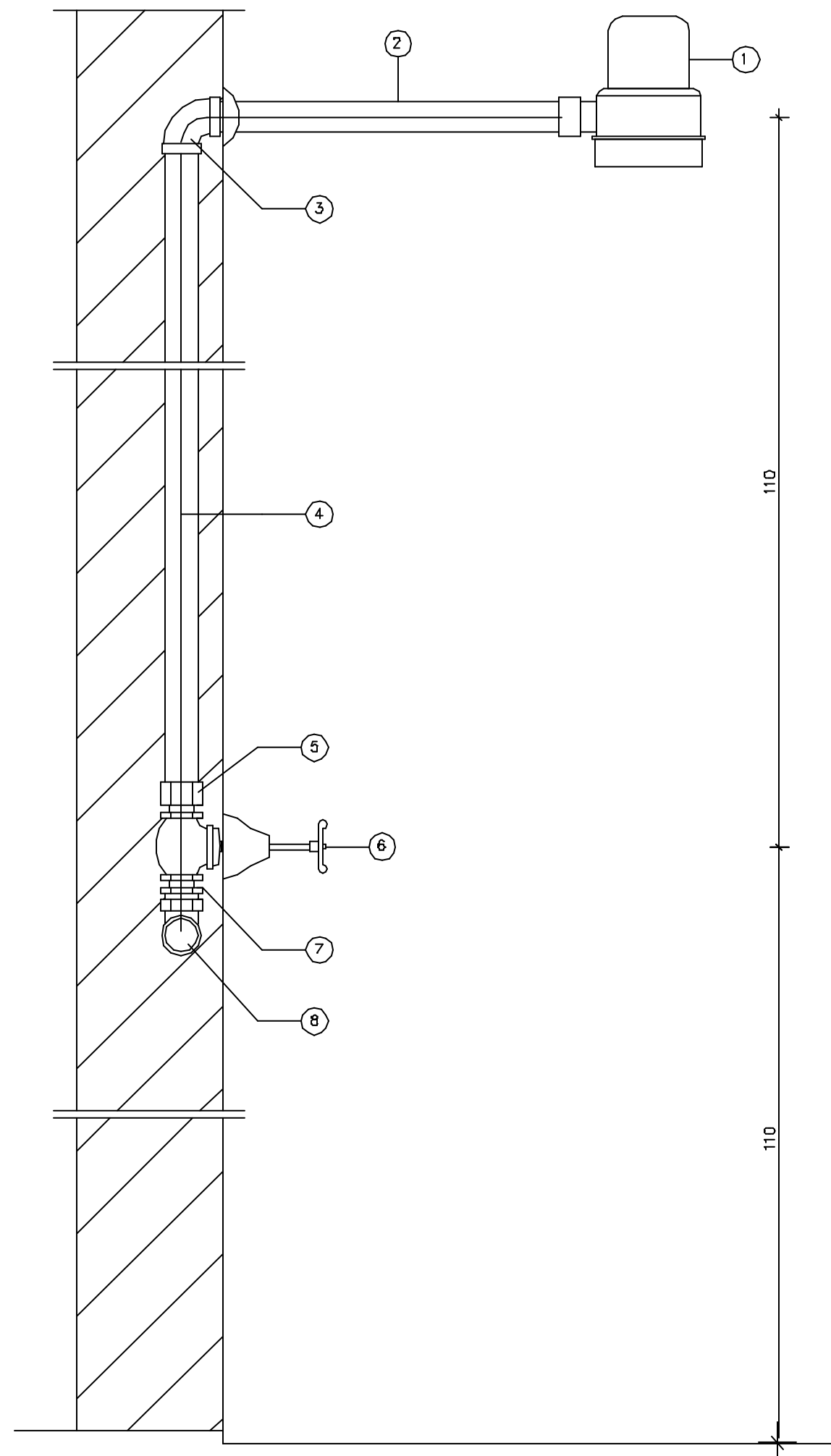
DETALHE INSTALACÃO DO CHUVEIRO
