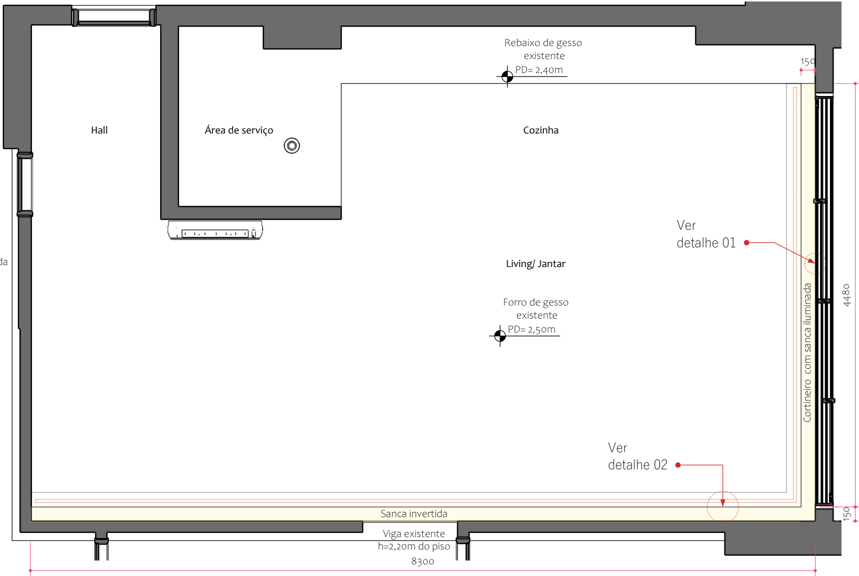
Planta de forro Esc.: 1/40
