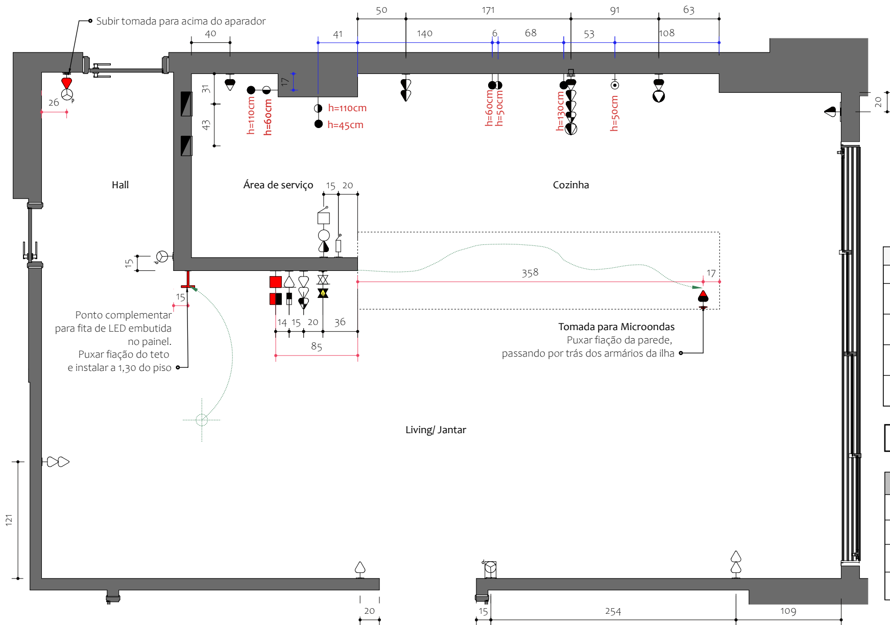
Planta pontos elétricos Esc.: 1/40
