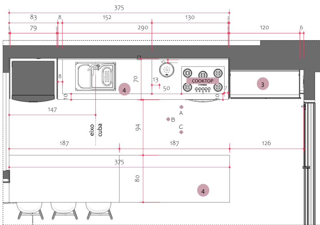
Planta baixa Esc.: 1/40
