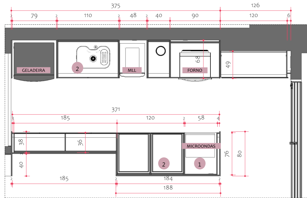
Planta baixa Esc.: 1/40
