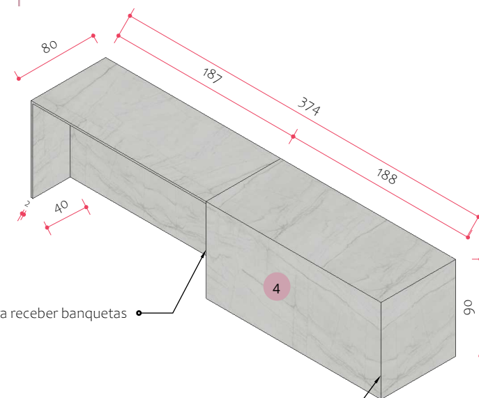
Detalhe Ilha Esc.: 1/40
