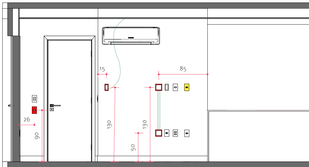
Vista A- Pontos elétricos Esc.: 1/40
