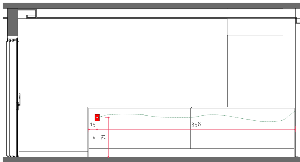
Vista B- Pontos elétricos Esc.: 1/40
