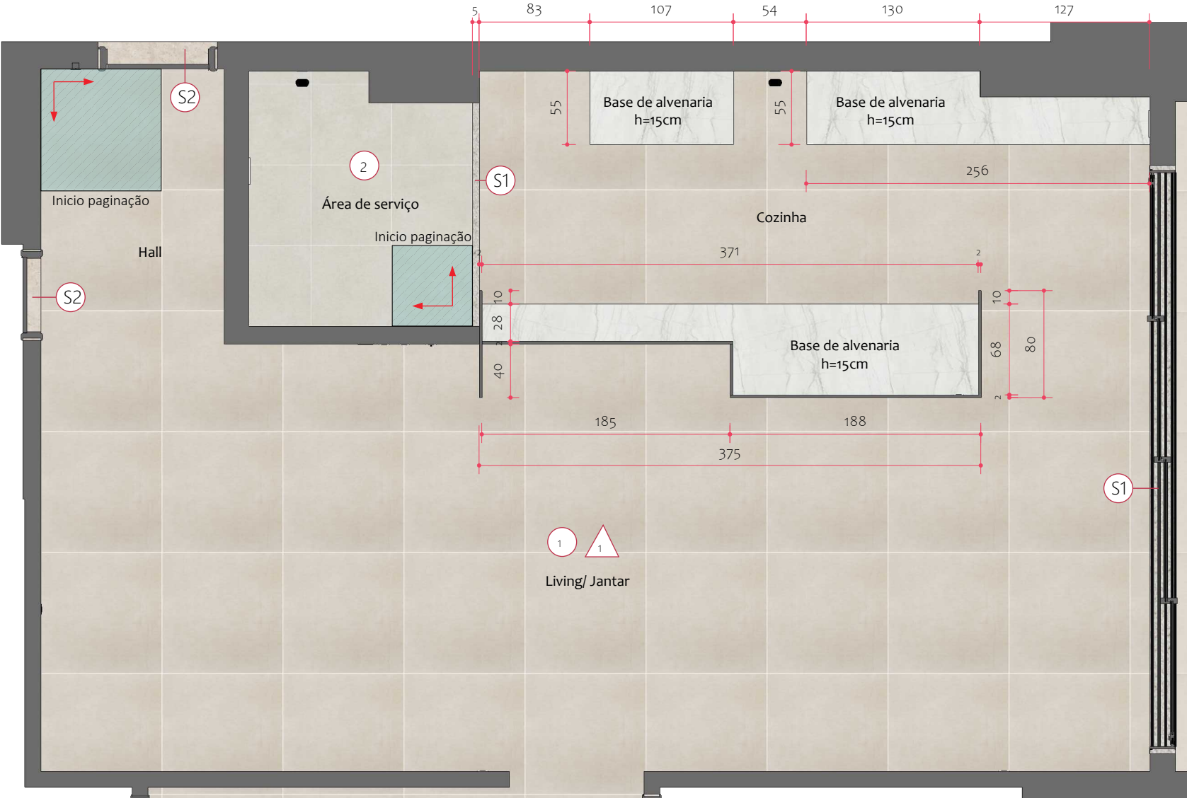
Planta de piso Esc.: 1/40
