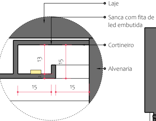
Detalhe 01- Cortineiro com sanca Esc.: 1/10
