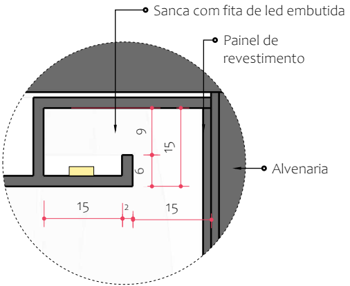
Detalhe 02- Sanca invertida Esc.: 1/10
