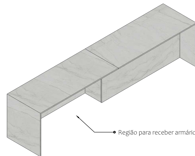
Detalhe Ilha Esc.: 1/40
