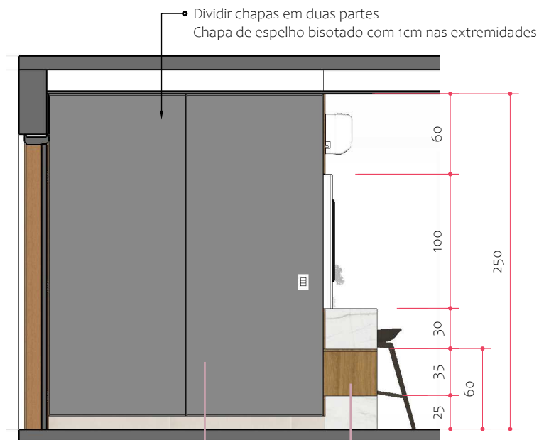
Vista C Esc.: 1/40
