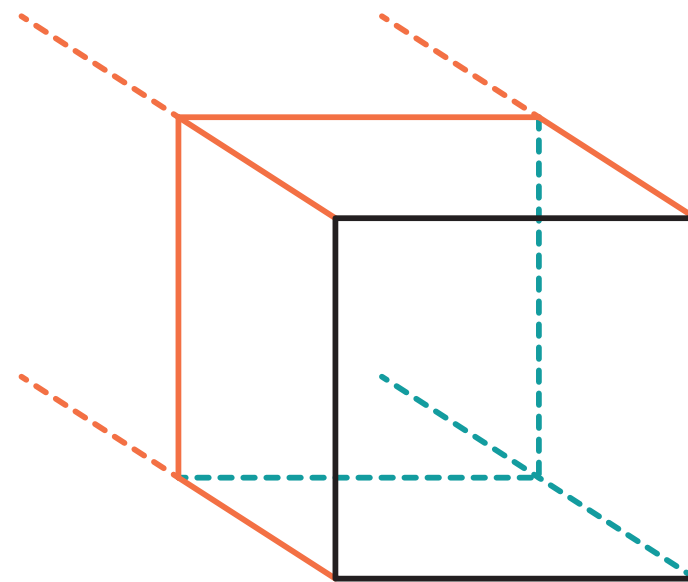
Perspectiva Cavaleira
