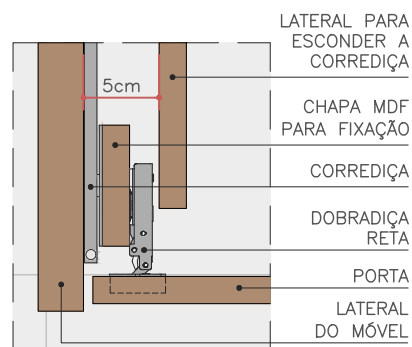
DET. FECHADO
