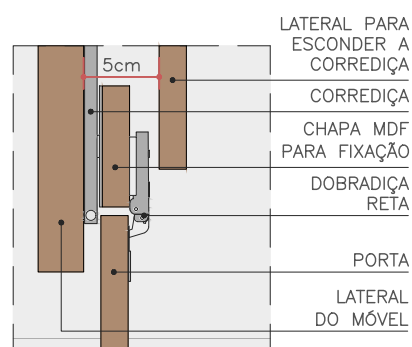
DET. ABERTO 1
