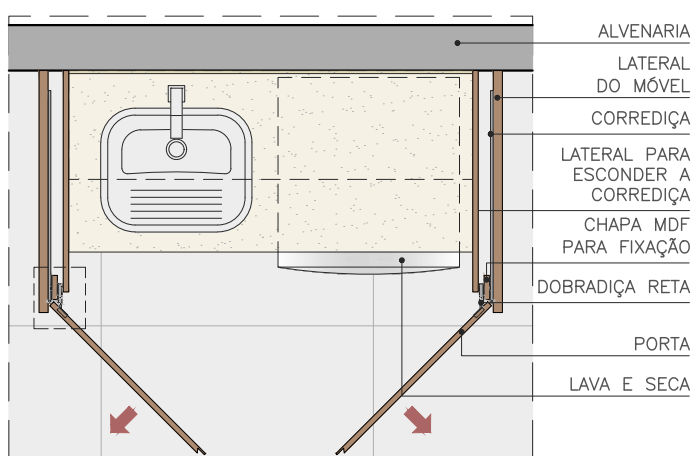
PLANTA ABERTURA 45°
