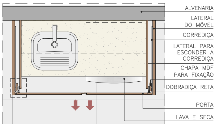
PLANTA FECHADO
