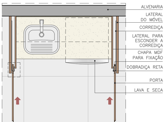
PLANTA ABERTO 1
