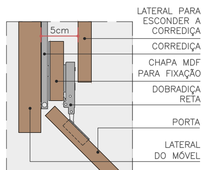
DET. ABERTURA 45°
