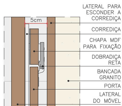
DET. ABERTO 3 ESC. 1:5
