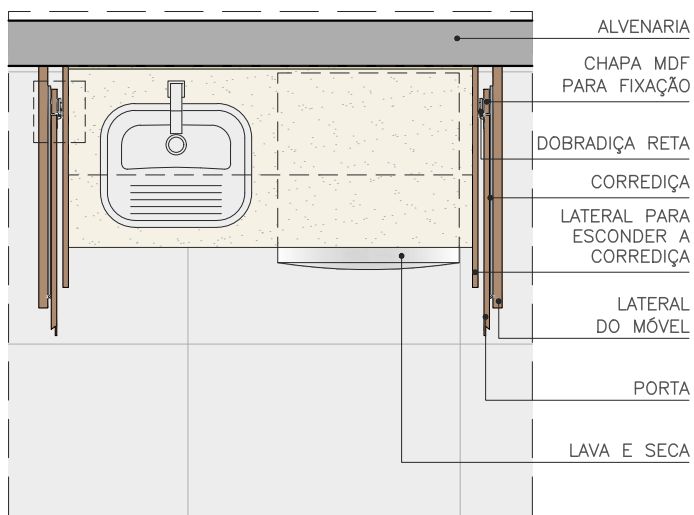
PLANTA ABERTO 3 ESC. 1:25
