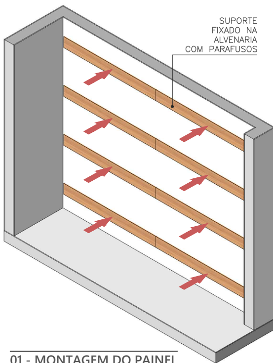
01 - MONTAGEM DO PAINEL SEM ESCALA
