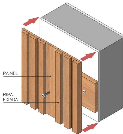
FIXAÇÃO DO PAINEL SEM ESCALA
