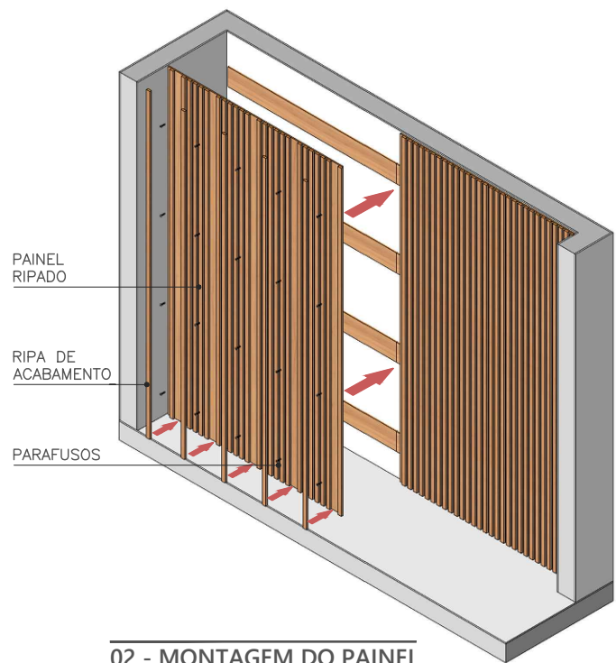
02 - MONTAGEM DO PAINEL SEM ESCALA
