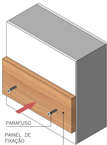
FIXAÇÃO DO SUPORTE SEM ESCALA
