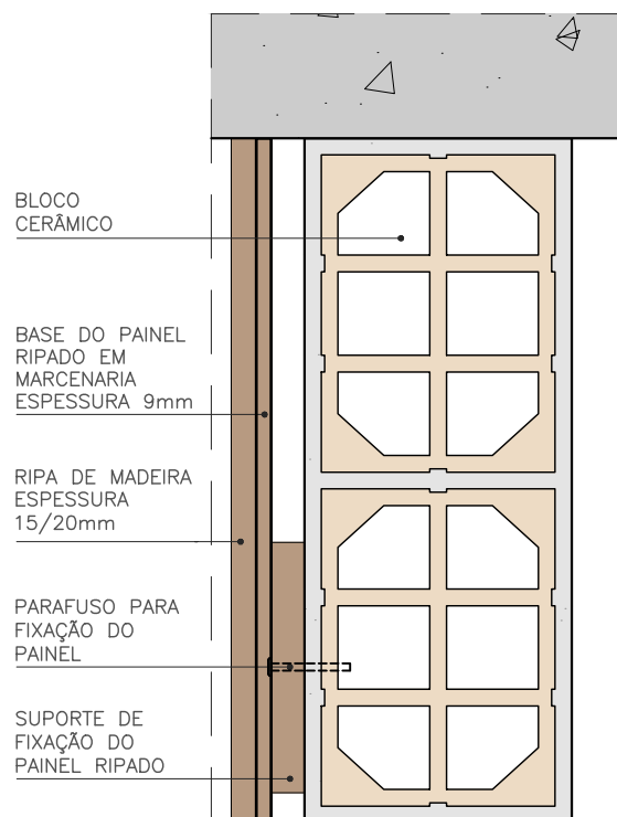
DET. CORTE
