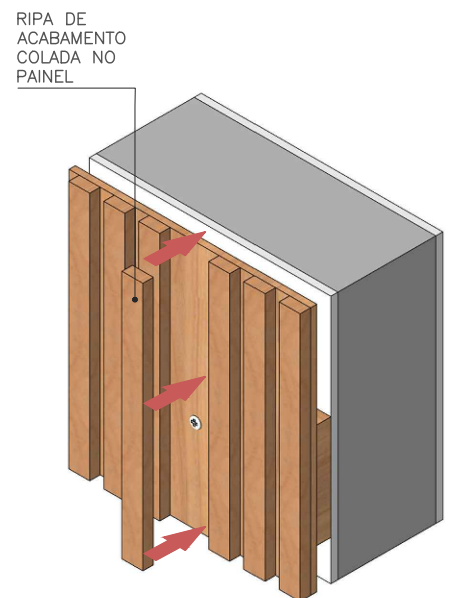
FIXAÇÃO DA RIPA DE ACABAMENTO SEM ESCALA
