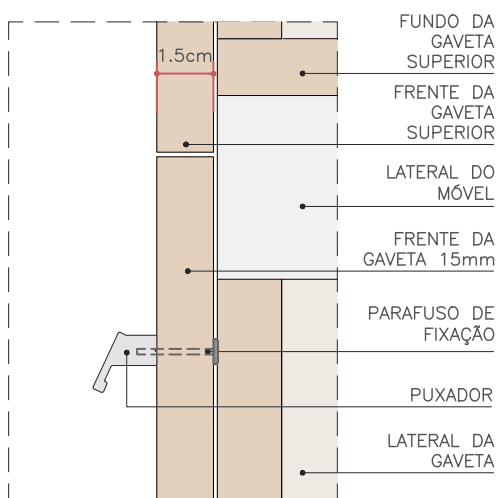
GAVETEIRO ESC. 1:2
