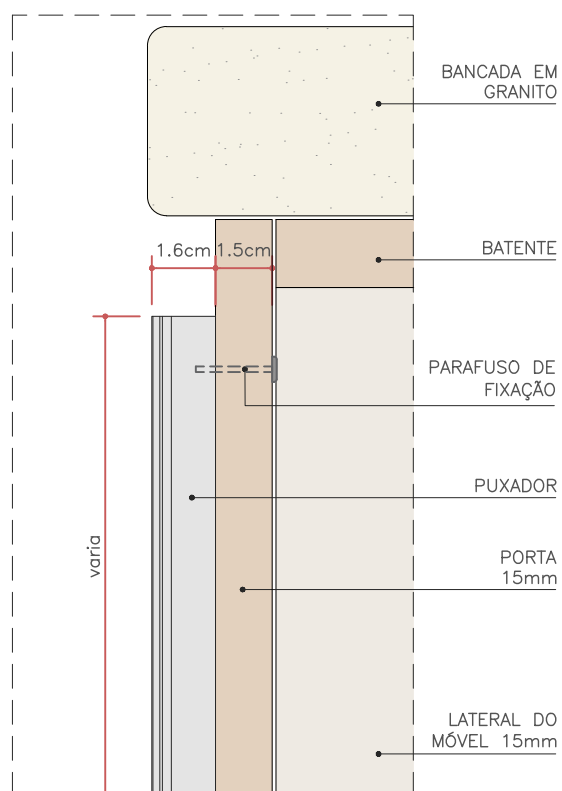
INFERIORES ESC. 1:2
