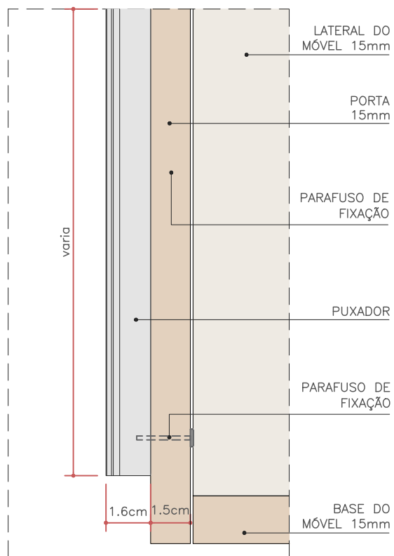
SUPERIORES ESC. 1:2
