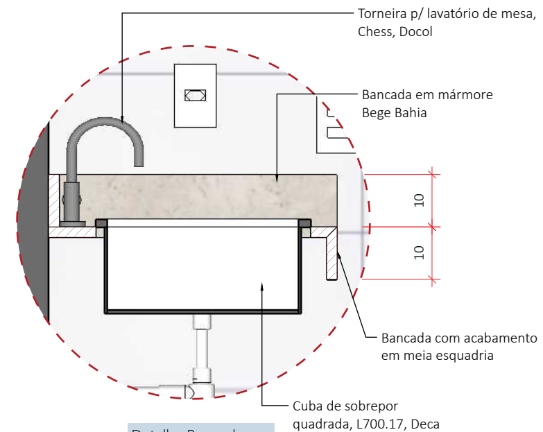
Detalhe Bancada
