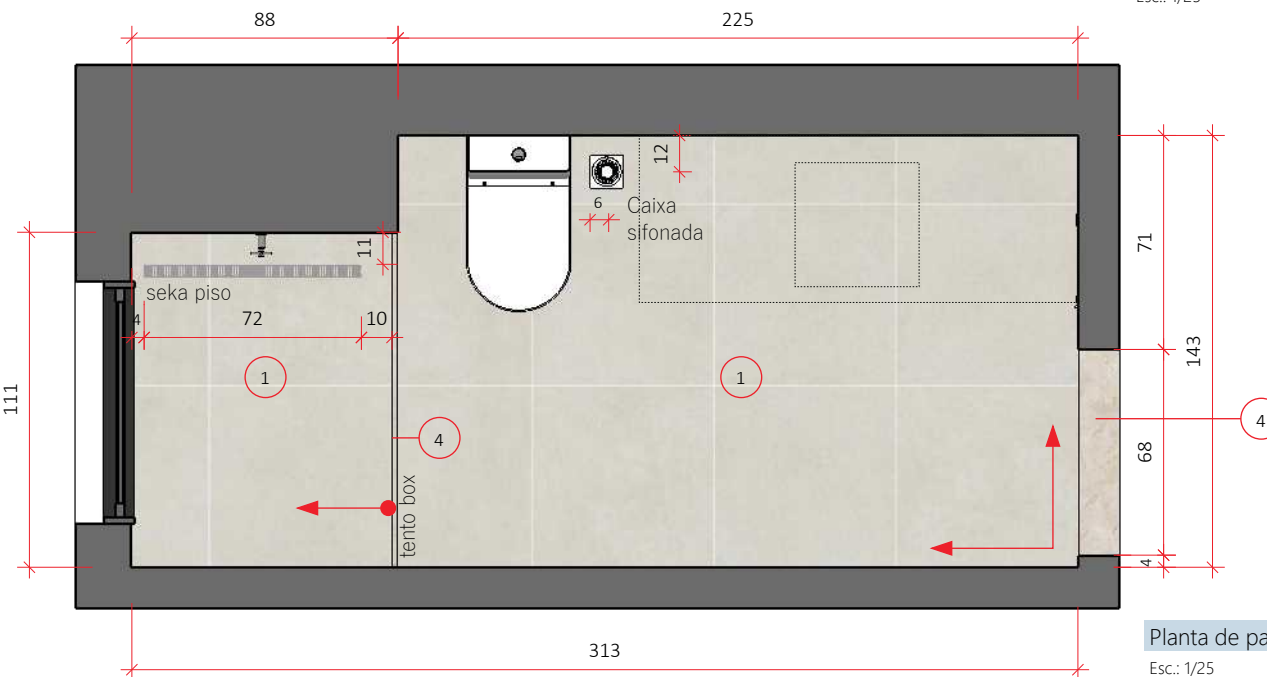
Planta Baixa
