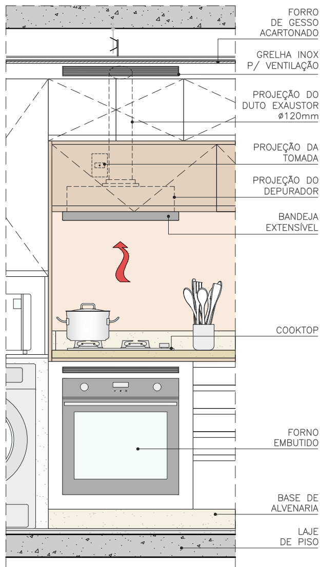
VISTA FRONTAL ESC. 1:20
