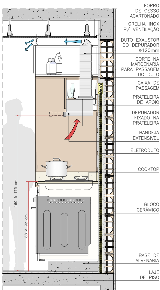
CORTE ESC. 1:20
