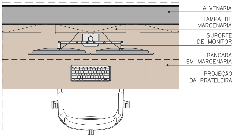
PLANTA ESC. 1:20
