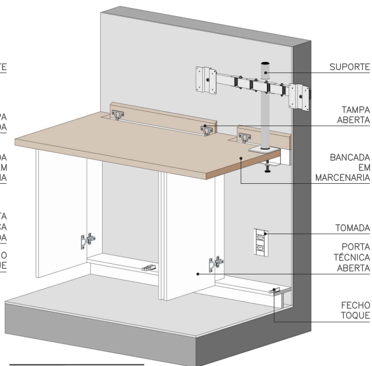
ISOMÉTRICA - ABERTA
