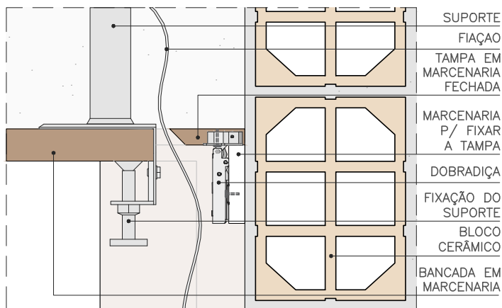
DET. CORTE - FECHADA
