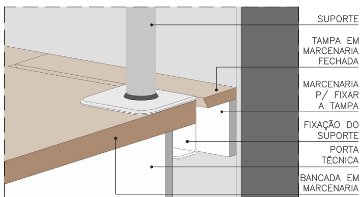
ISOMÉTRICA - FECHADA
