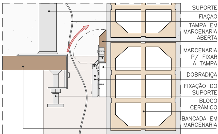
DET. CORTE - ABERTA
