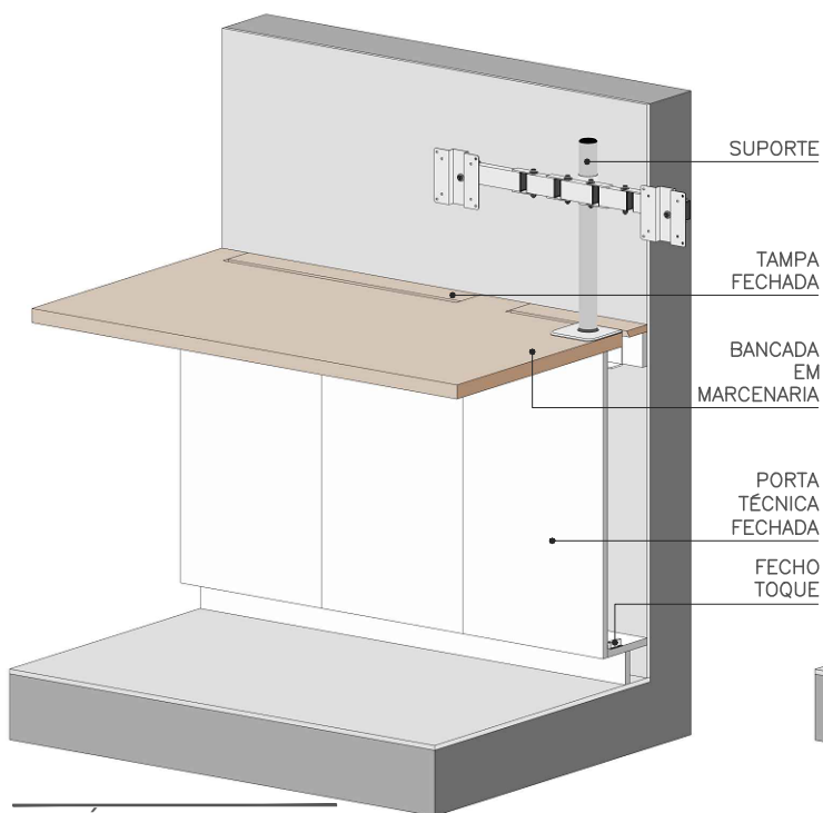
ISOMÉTRICA - FECHADA
