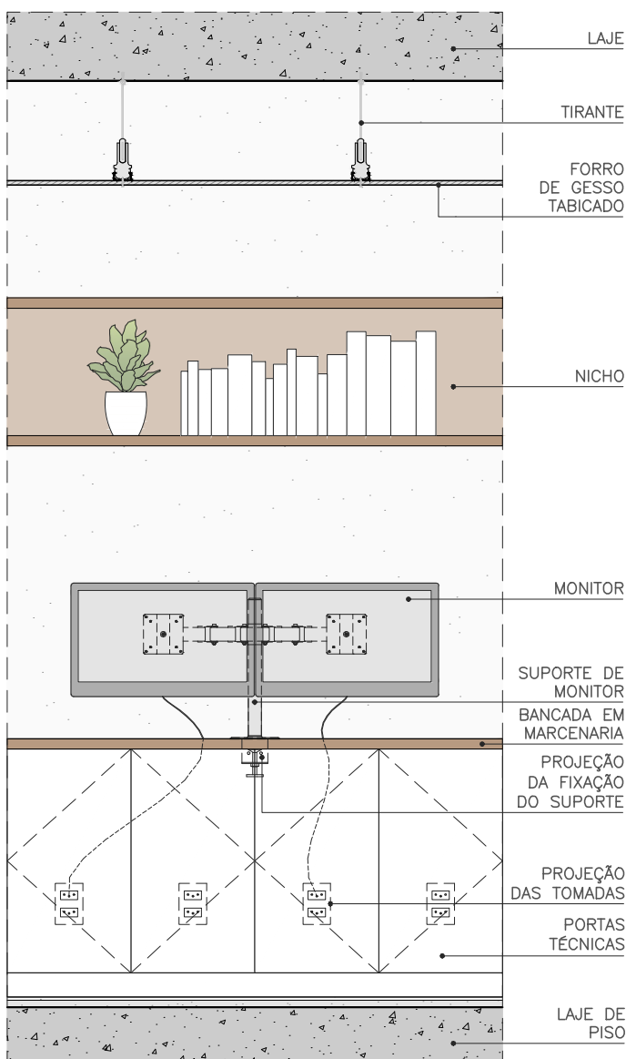
VISTA FRONTAL - FECHADA ESC. 1:20
