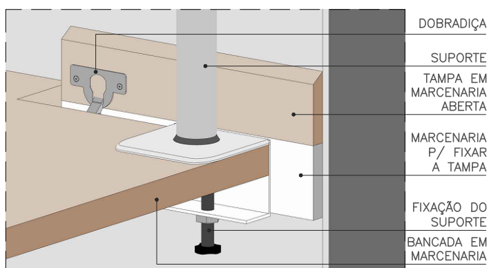
ISOMÉTRICA - ABERTA
