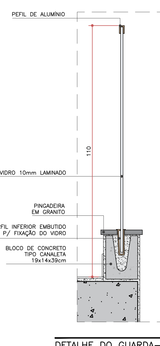
DETALHE DO GUARDA-CORPO DA PASSARELA E ESCALADA EXTERNA ESC. 1:10
