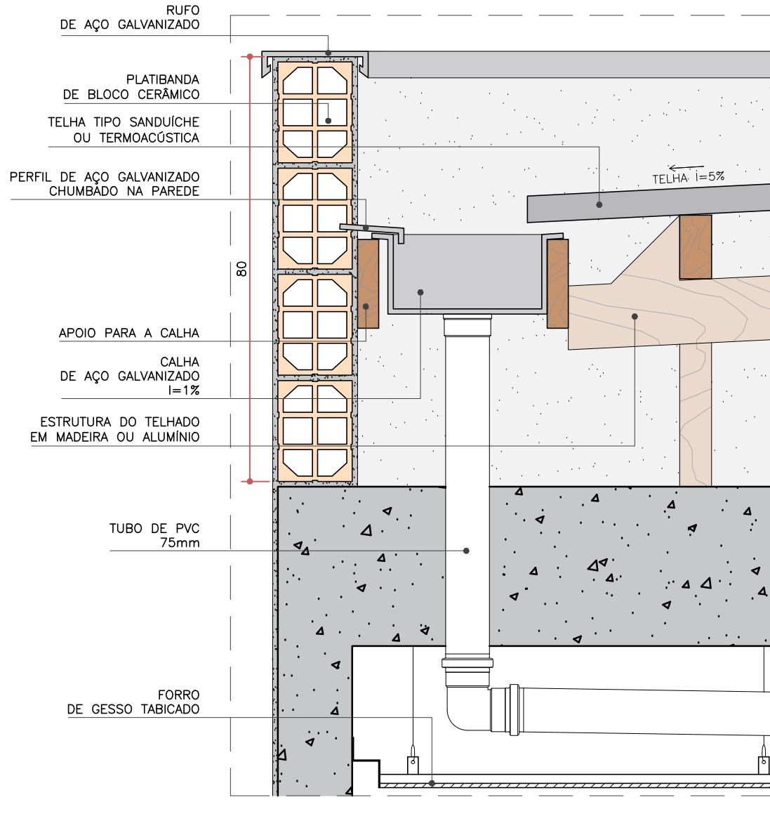
DETALHE DA PLATIBANDA ESC. 1:10
