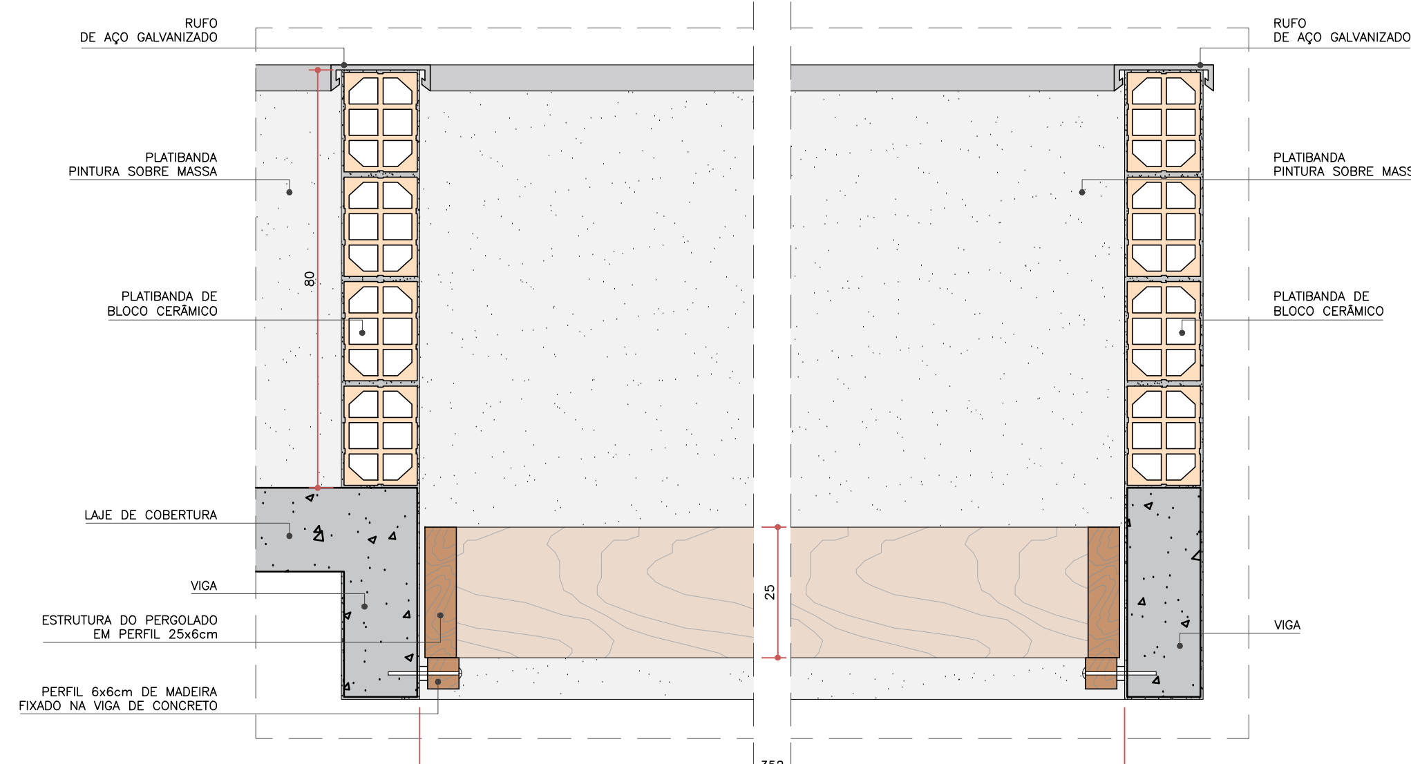
DETALHE DO PERGOLADO DA GARAGEM ESC. 1:10
