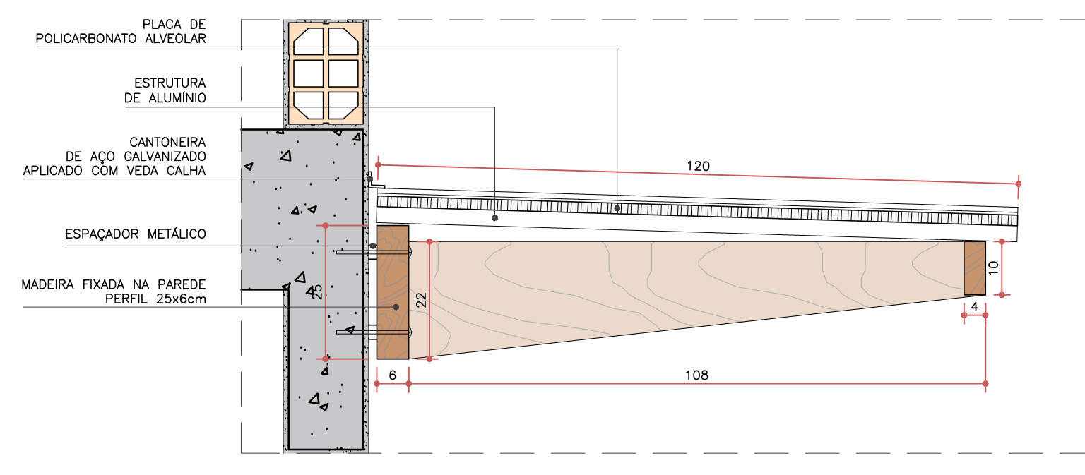
DETALHE DO PERGOLADO DA PASSARELA ESC. 1:10
