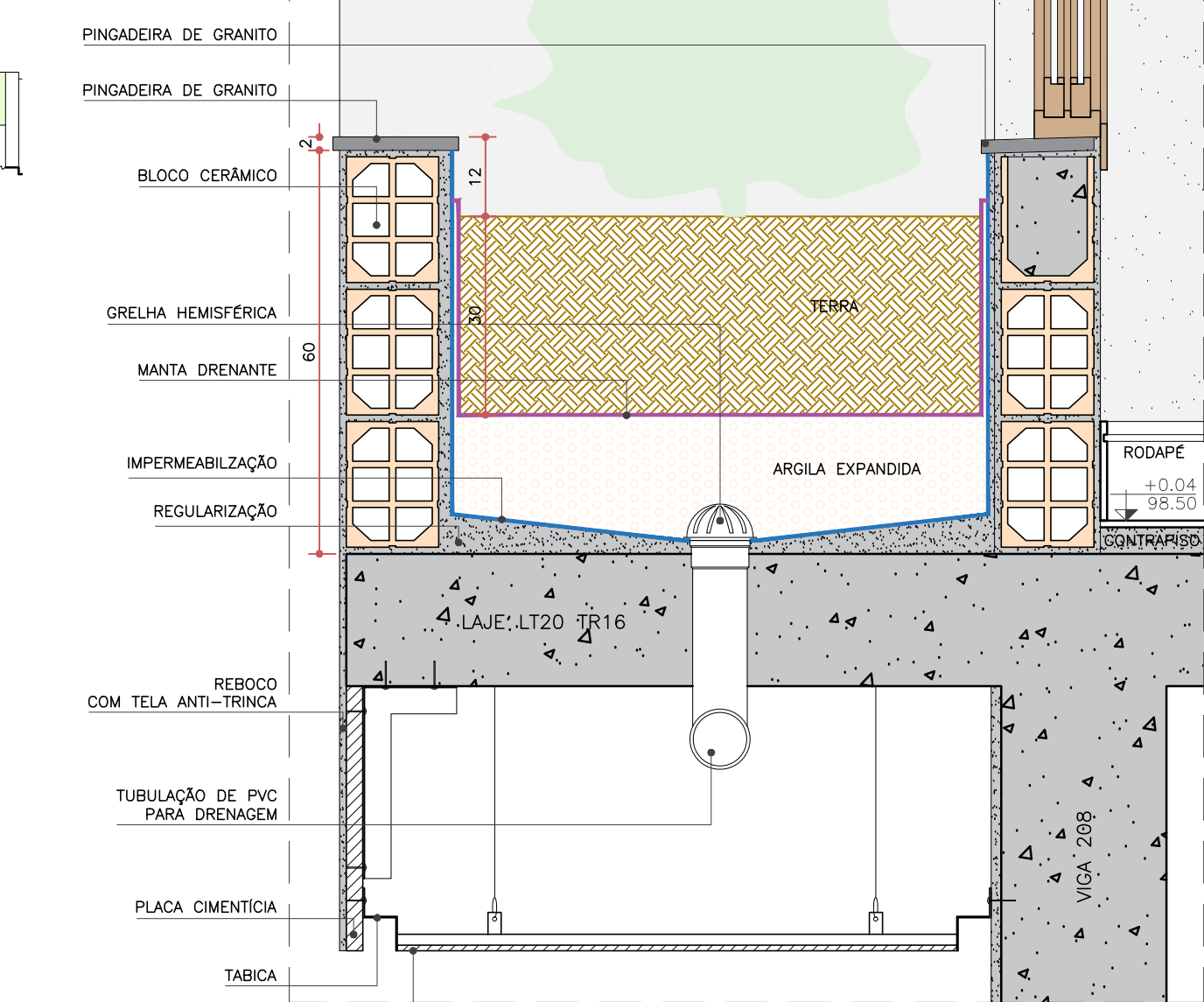
DETALHE DA JARDINEIRA + BEIRAL DA COBERTURA ESC. 1:10
