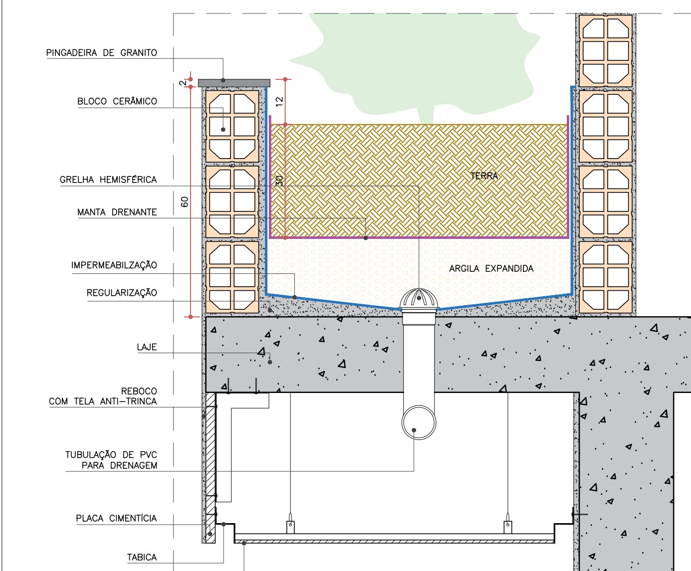
DETALHE DA JARDINEIRA (CORTE A) ESC. 1:10
