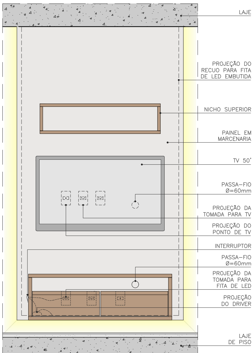
VISTA FRONTAL ESC. 1:20
