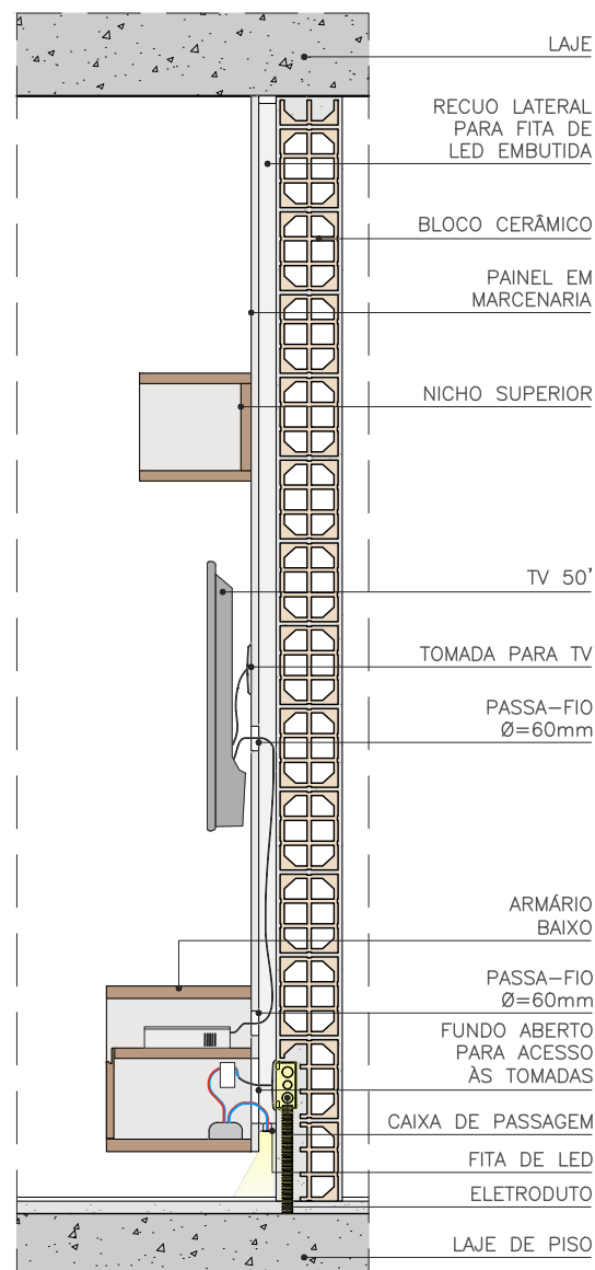
CORTE ESC. 1:20
