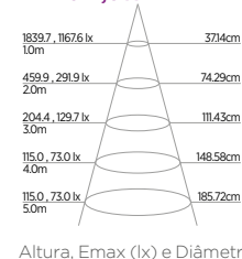
Gráfico 1 – Lâmpada AR70 4,8W
