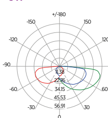
Gráfico 3 – Balizador 3W
