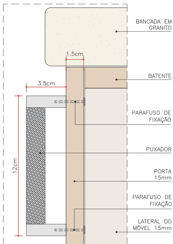
INFERIORES ESC. 1:2
