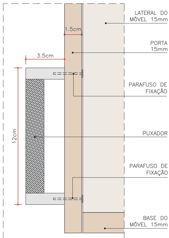
SUPERIORES ESC. 1:2
