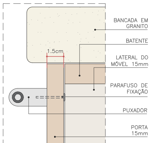
INFERIORES ESC. 1:2
